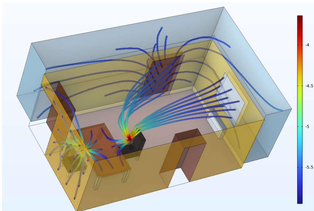
Рисунок 21 – Распространение потока энергии в дБ
