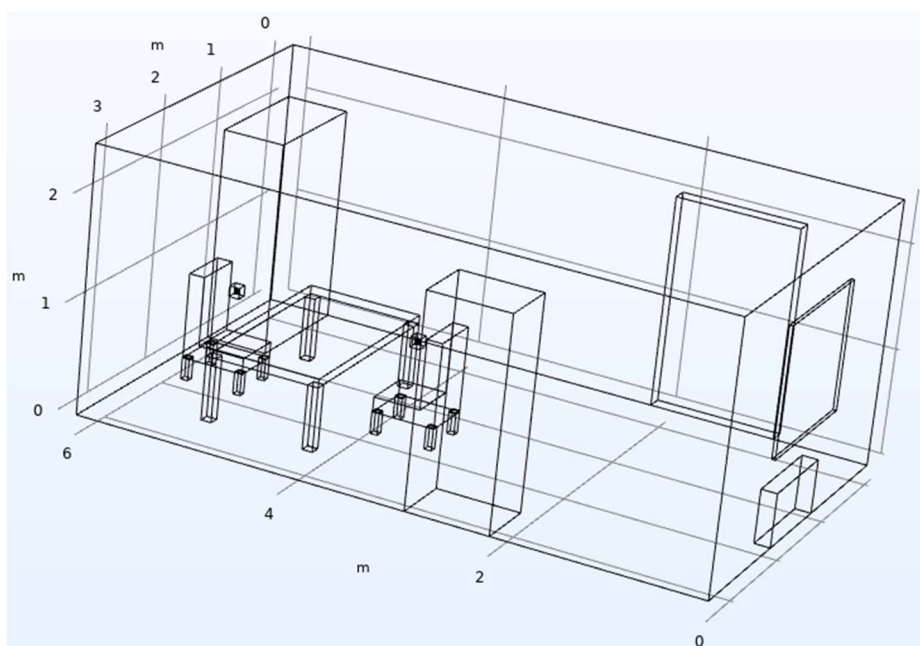
Рисунок 8 – Итоговая геометрия исследуемого помещения в пространстве
