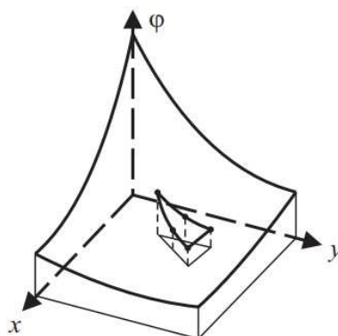
Рисунок 6 – Элемент с пятью узловыми точками
