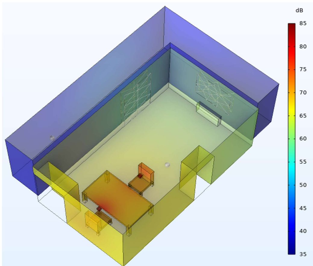
Рисунок 20 – Распространение звукового давления в дБ
