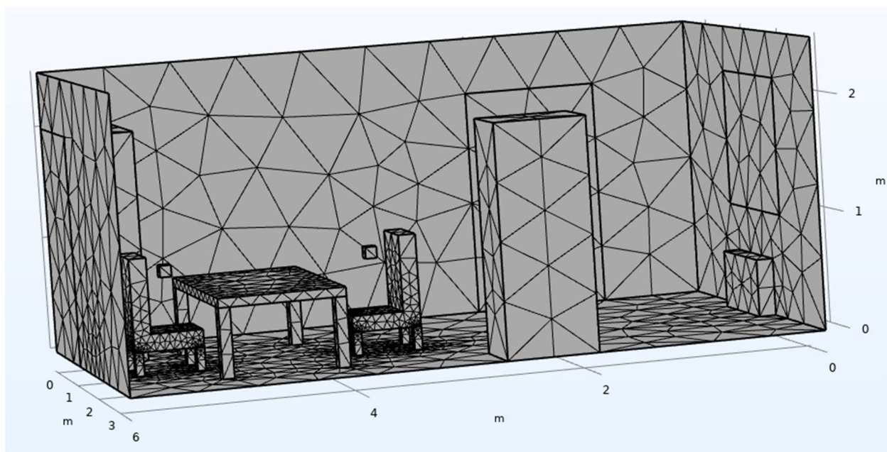
Рисунок 19 – Модель, разбитая на конечные элементы
