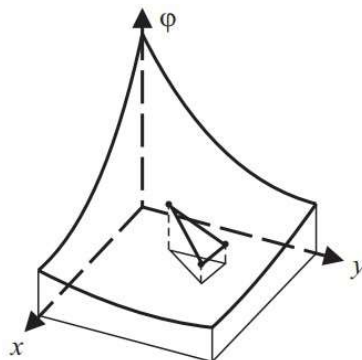
Рисунок 5 – Элемент с треугольной формой, состоящий из трёх узлов
