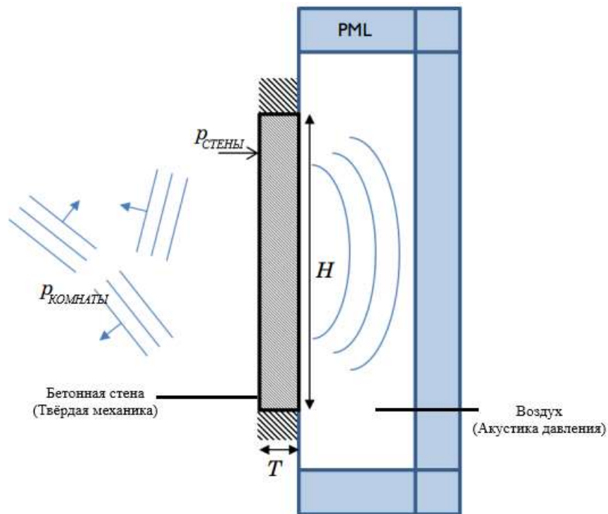
Рисунок 23 – Модель рассматриваемой бетонной стены
