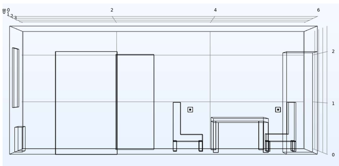
Рисунок 10 – Итоговая геометрия исследуемого помещения относительно осей XZ
