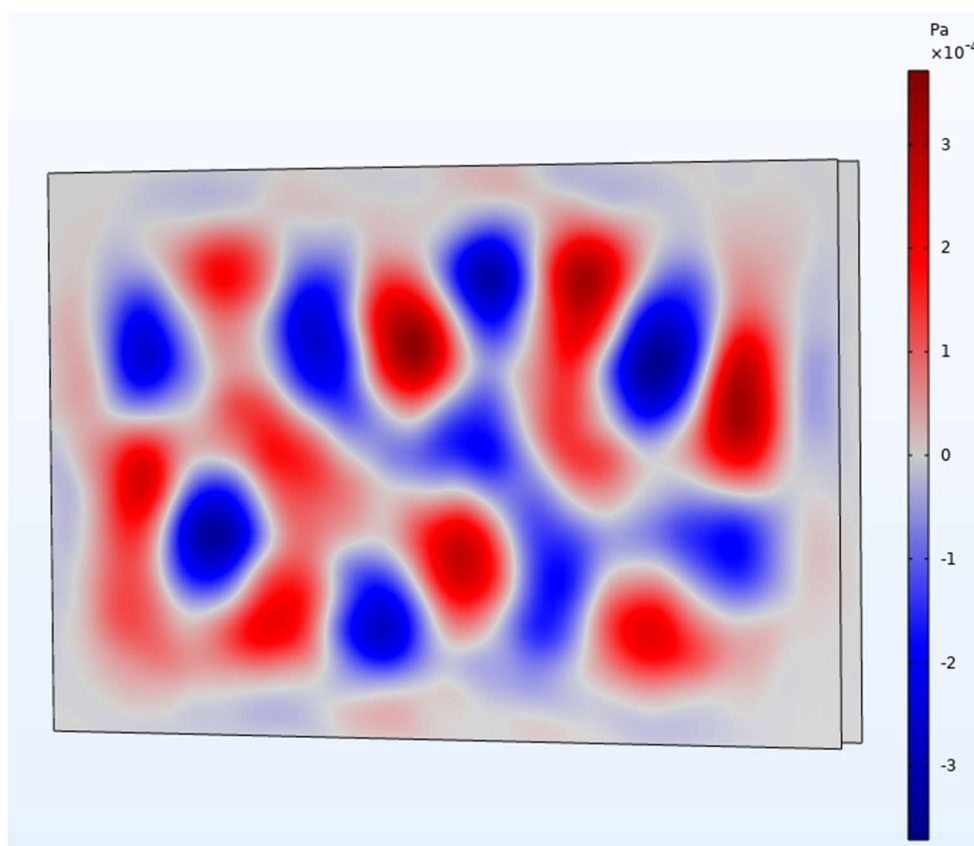
Рисунок 25 – Общее акустическое давление сквозь стену
