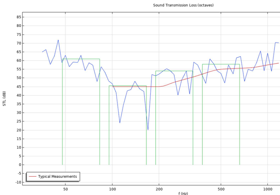
Рисунок 26 – Расчётные потери на передачу звука (STL)
