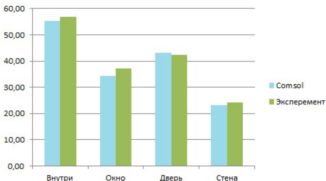
Рисунок 22 – Сравнение показателей замеров и моделирования в «Comsol»
