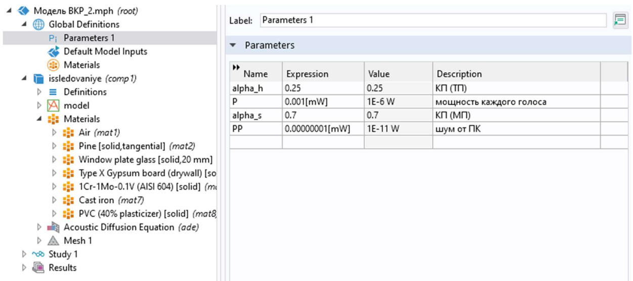
Рисунок 11 – Глобальные параметры
