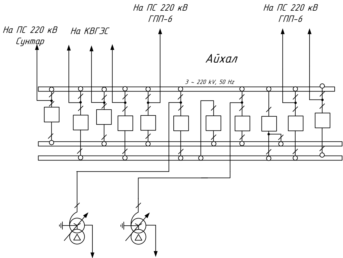
Рисунок 19 – Распределительное устройство 220 кВ подстанции Айхал
