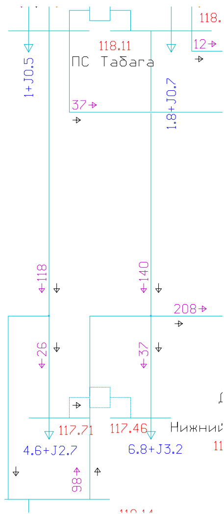
Рисунок 20 – определение расчетного тока по ВЛ 110 кВ Табага – Майя № 2
