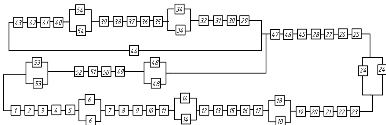
Рисунок 30 – Схема замещения для расчета надежности
