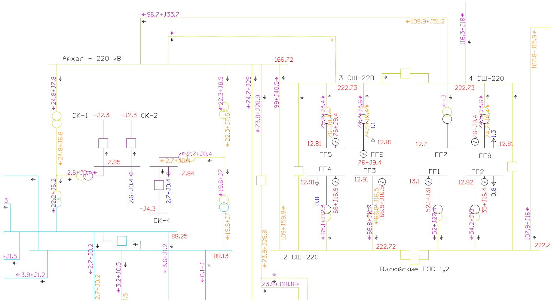
Рисунок 6 – Аварийное отключение ВЛ 220 кВ Виллюйская ГЭС – Айхал в нормальной схеме
