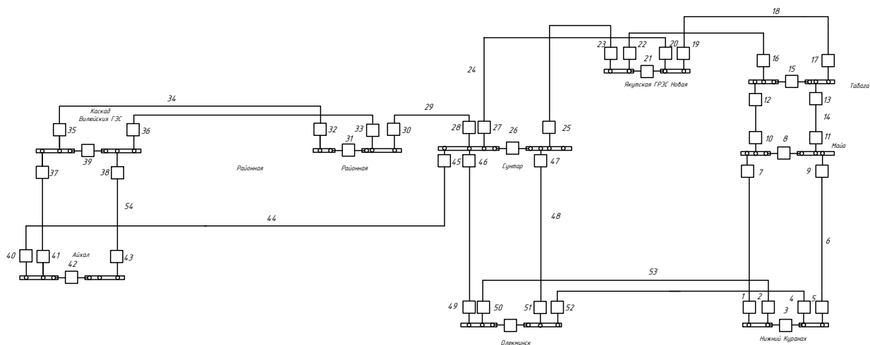
Рисунок 29 – Схема объединения энергосистем
