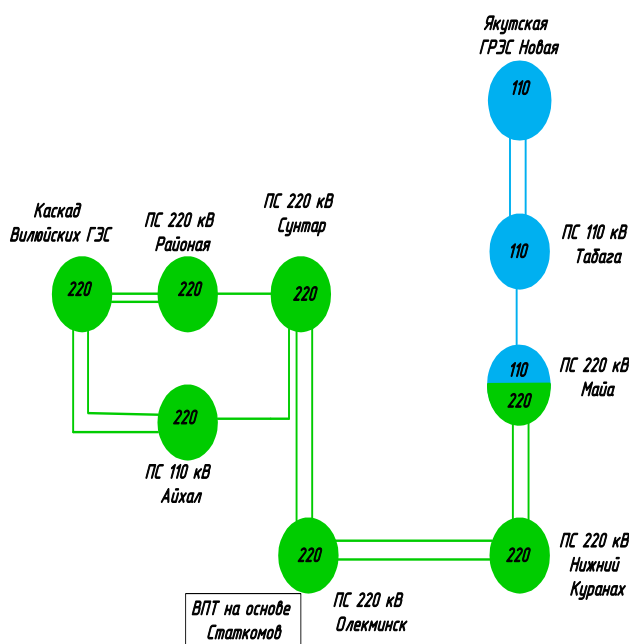
Рисунок 13 – Структурная схема объединения с помощью ВЛ 500 кВ
