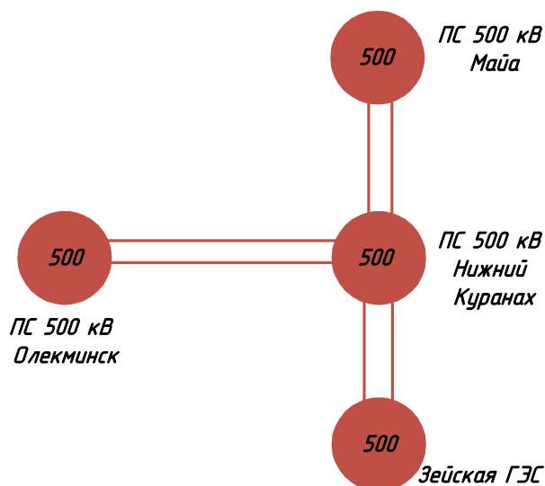
Рисунок 12 – Структурная схема объединения с помощью ВЛ 500 кВ
