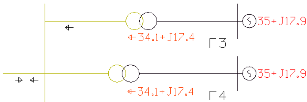
Рисунок 16 – Переток мощности по блочным трансформаторам Якутской ГРЭС Новой
