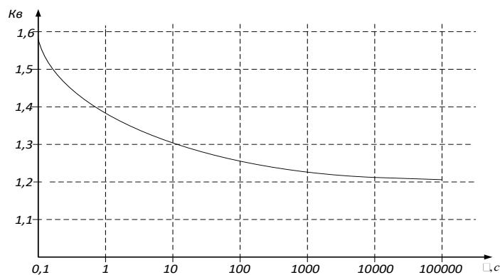
Рисунок 17 – График зависимости коэффициента K_B от длительности
