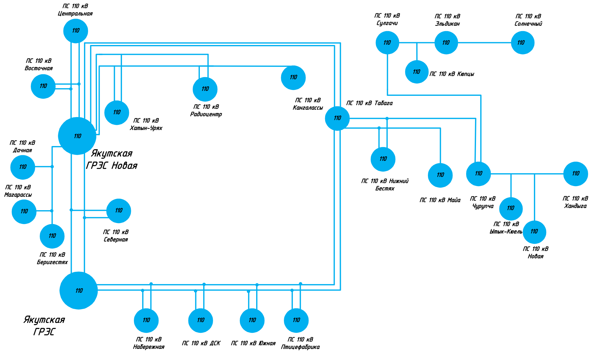
Рисунок 3 – Граф электрической сети Центрального энергорайона Республики Саха (Якутия)
