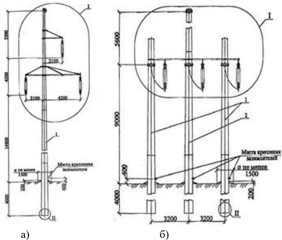
Рисунок 22 – Стальная многогранная промежуточная опора ВЛ 110 кВ (а), стальная анкерно-угловая опора ВЛ 110 кВ (б)
