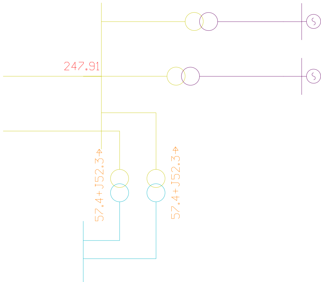
Рисунок 15 – Гереток мощности по силовым трансформаторам на Якутской ГРЭС Новой
