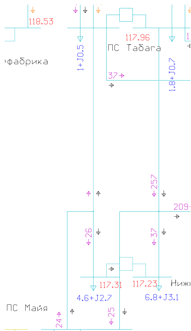
Рисунок 21 – Определение расчетного тока в послеаварийном режиме по ВЛ 110 кВ Табага – Майя № 2
