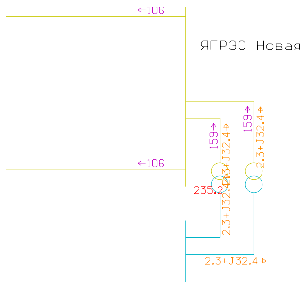
Рисунок 23 – Определение расчетного тока в нормальном режиме по ВЛ 220 кВ Якутская ГРЭС Новая – Сунтар № 1 и № 2
