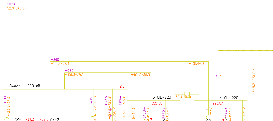
Рисунок 27 – Расчетный ток по ВЛ 220 кВ Сунтар – Айхал в послеаварийном режиме
