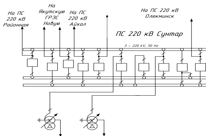
Рисунок 19 – Распределительное устройство 220 кВ подстанции Сунтар
