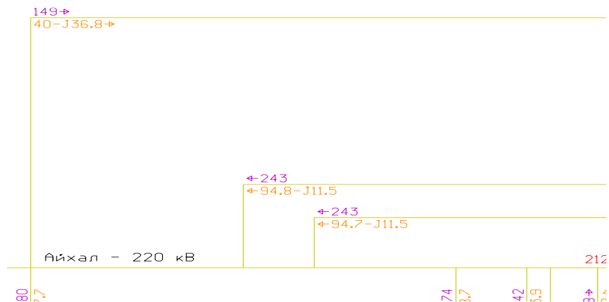
Рисунок 26 – Расчетный ток по ВЛ 220 кВ Сунтар – Айхал в нормальном режиме
