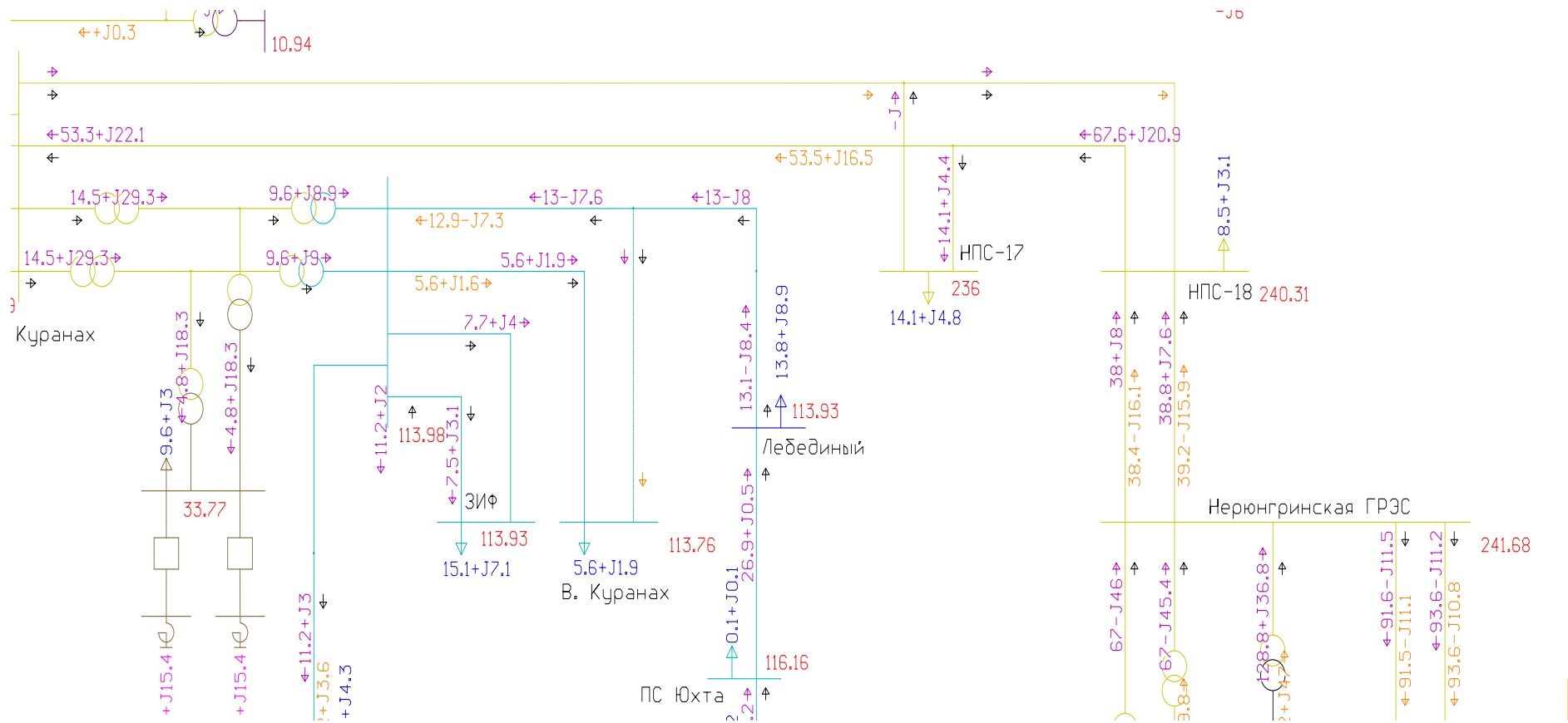
Рисунок 9 – Аварийное отключение ВЛ 220 кВ Нижний Куранах – НПС-18 № 2 с отпайкой на ПС НПС-17 в нормальной схеме
