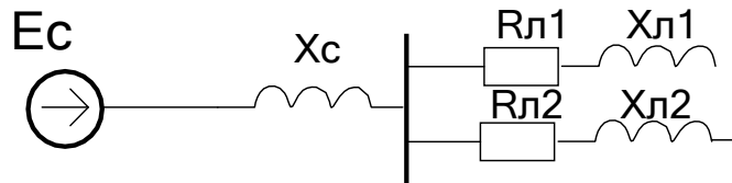
Рисунок 7 – Расчетная схема замещения короткого замыкания на 10 кВ
