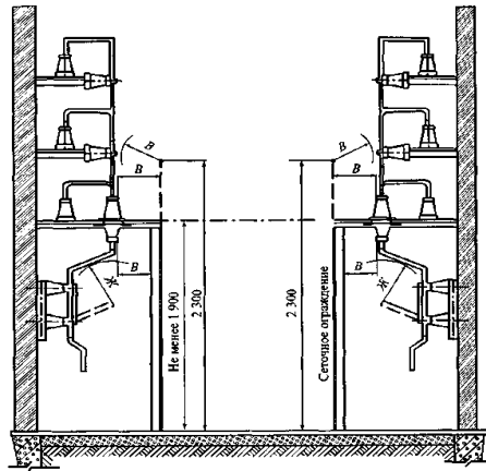
Рисунок 14 - Наименьшие расстояния от неизолированных токоведущих частей в ЗРУ до сетчатых ограждений и между неогражденными неизолированными токоведущими частями разных цепей
