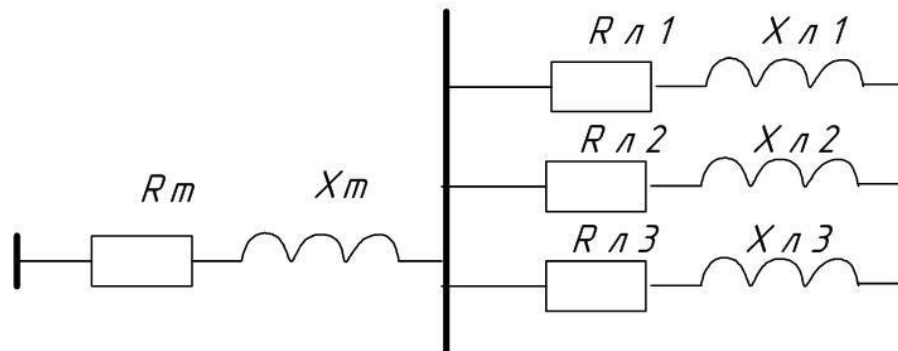
Рисунок 4 – Расчетная схема
