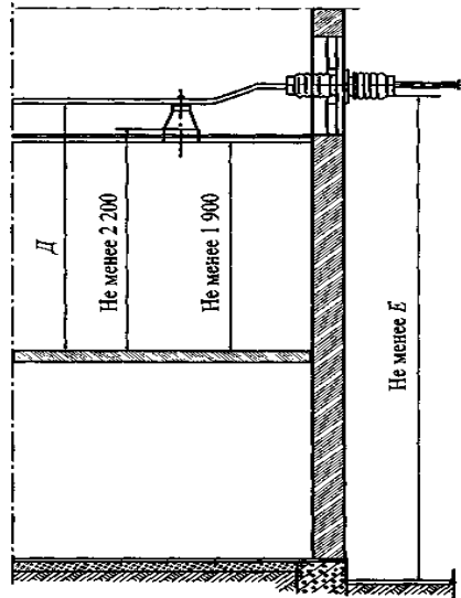
Рисунок 15 - Наименьшие расстояния от пола до неогражденных неизолированных токоведущих частей и до нижней кромки фарфора изолятора и высота прохода в ЗРУ. Наименьшее расстояние от земли до неогражденных линейных выводов из ЗРУ вне территории ОРУ и при отсутствии проезда транспорта под выводами.
