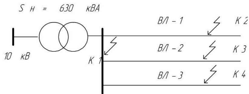
Рисунок 4 – Расчетная схема
