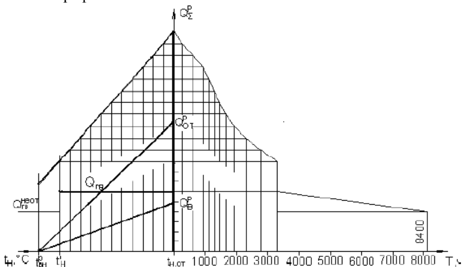
Рисунок 1 - Расчетный и годовые расходы теплоты в горячей воде
