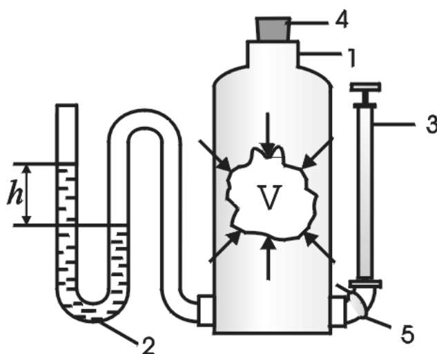
Рис. 1. Схема установки.
