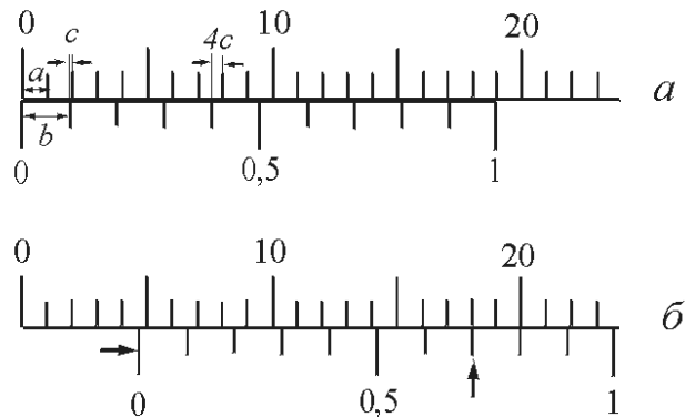
Рис. 2. Устройство нониуса ( \lambda = 2 , c = 0,1 ).
