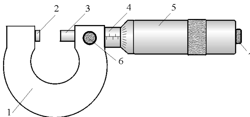
Рис 3. Устройство микрометра.
