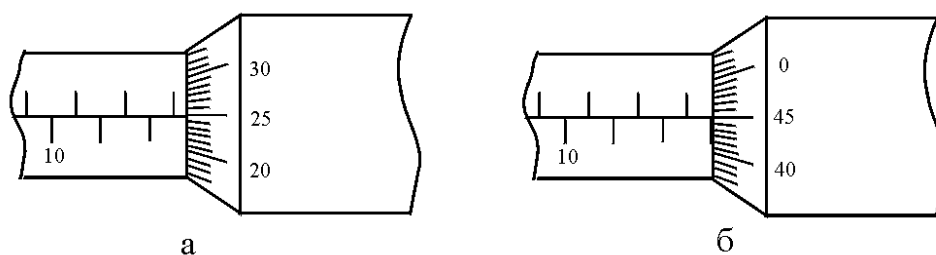
Рис.4. Отсчетное устройство микрометра;
