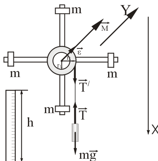
Рис.1. Схема установки.
