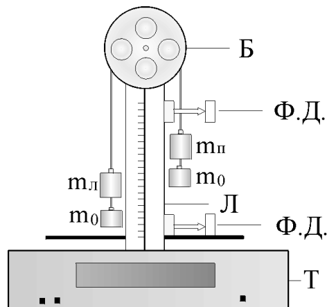
Рис. 2 . Схема экспериментальной установки: m_n, m_n - основные грузы; m_o - перегрузки ; B - блок ; T - миллисекундомер; L - линейка, \Phi Д - фотоэлектрические датчики.
