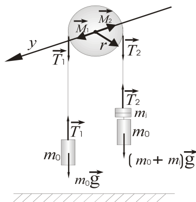
Рис.3. Учет инерции блока.
