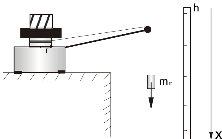
Рис.2. Схема установки.
