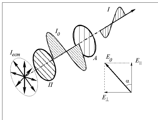
Рис. 2 Схема прохождения световой волны через систему поляризатора и анализатора.
