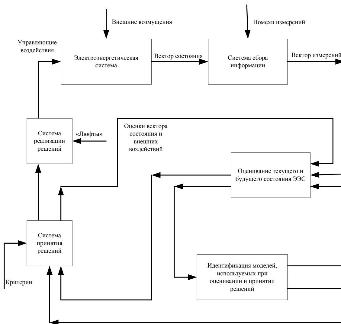
Рис. 3.3. Схема обработки информации при управлении ЭЭС
