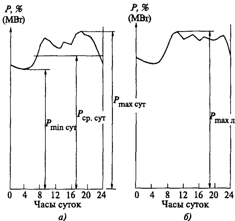
Рис. 2.6. Суточные графики электрических нагрузок: а) с вечерним максимум нагрузки; б) с одинаковым утренним и вечерним максимумами нагрузки
