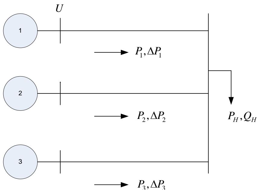
Рис. 4.1. Схема системы к выводу условия оптимального распределения нагрузки
