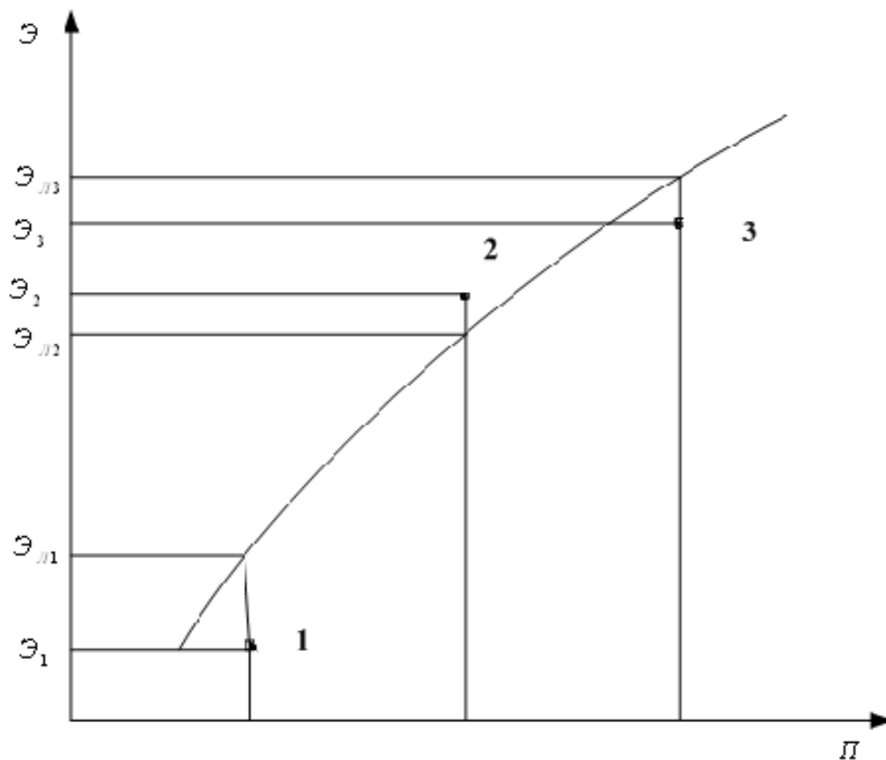
Рис. 2.4. Характеристика расхода электроэнергии \mathcal{E} на выпуск продукции \Pi
