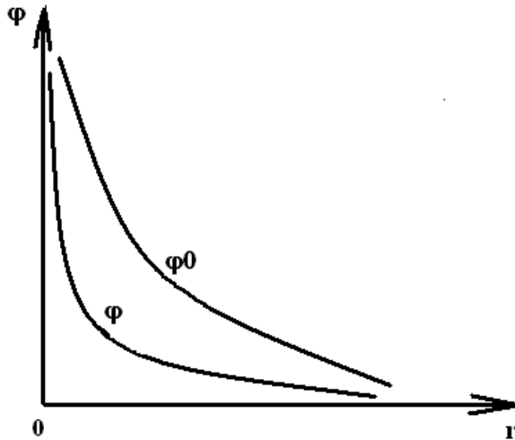
Рисунок 4 – Короткодействующее и далекодействующее поля
