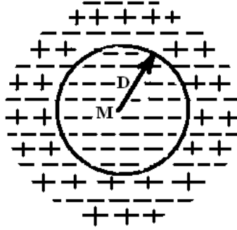
Рисунок 3 – Точечный заряд в ионизированном газе
