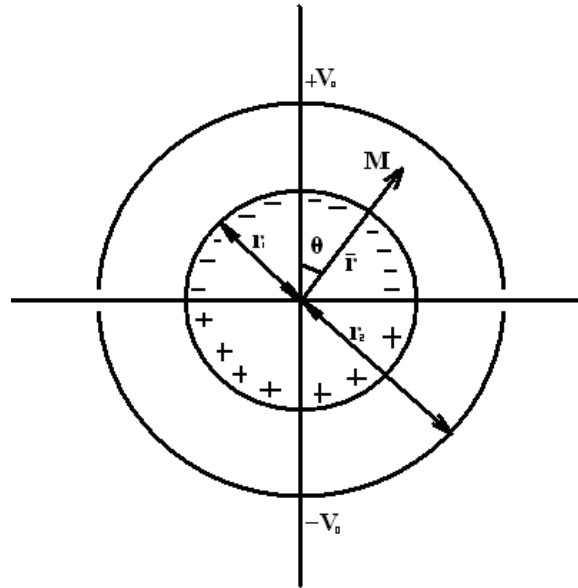
Рисунок 2 – Электростатический подвес
