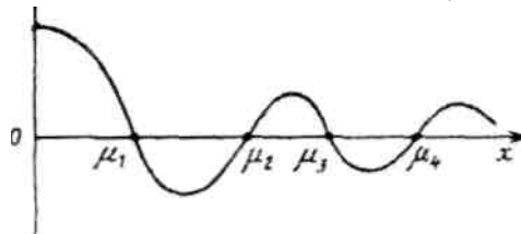
Рисунок 5 – График функции J_0(x)
