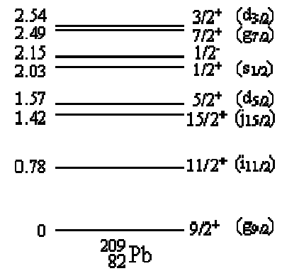
Рис. 4. Возбужденные уровни ^{209}\text{Pb}
