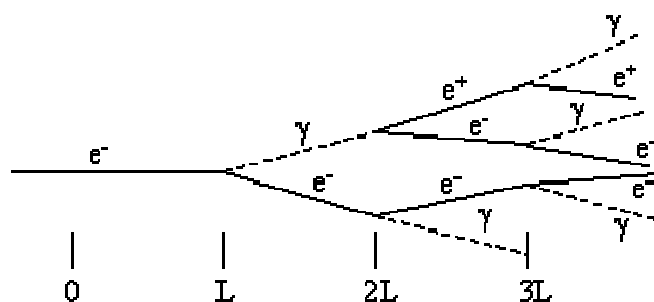
Рис. 4. Каскадный ливень
