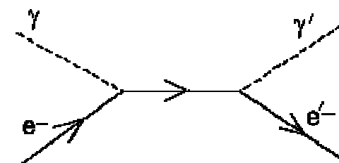
Рис.6. Эффект Комптона
