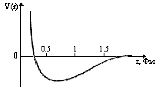
Нуклон-нуклонный потенциал
