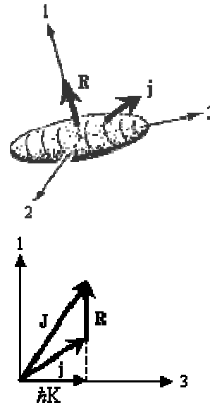
Рис. 6. Вращательные и одночастичные степени свободы. R - коллективный момент количества движения, j - одночастичный момент количества движения валентного нуклона, J - полный момент количества движения, \hbar K - собственное значение полного момента J вдоль оси симметрии 3
