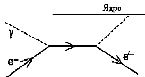
Рис. 5. Фотоэффект
