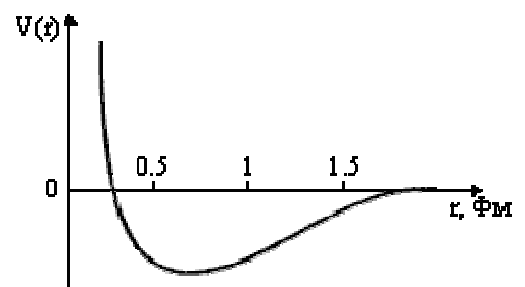
Рис. 4. Нуклон-нуклонный потенциал
