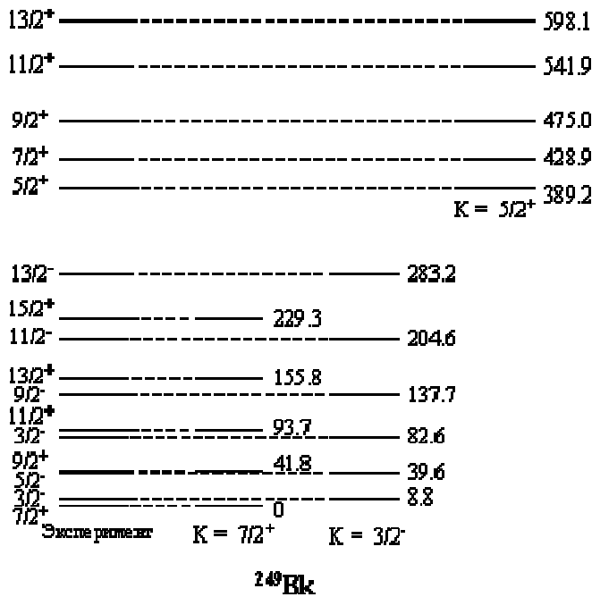
Рис. 7. Энергетические уровни 249 Bk. Справа выделены 3 вращательные полосы. Энергии уровней даны в кэВ
