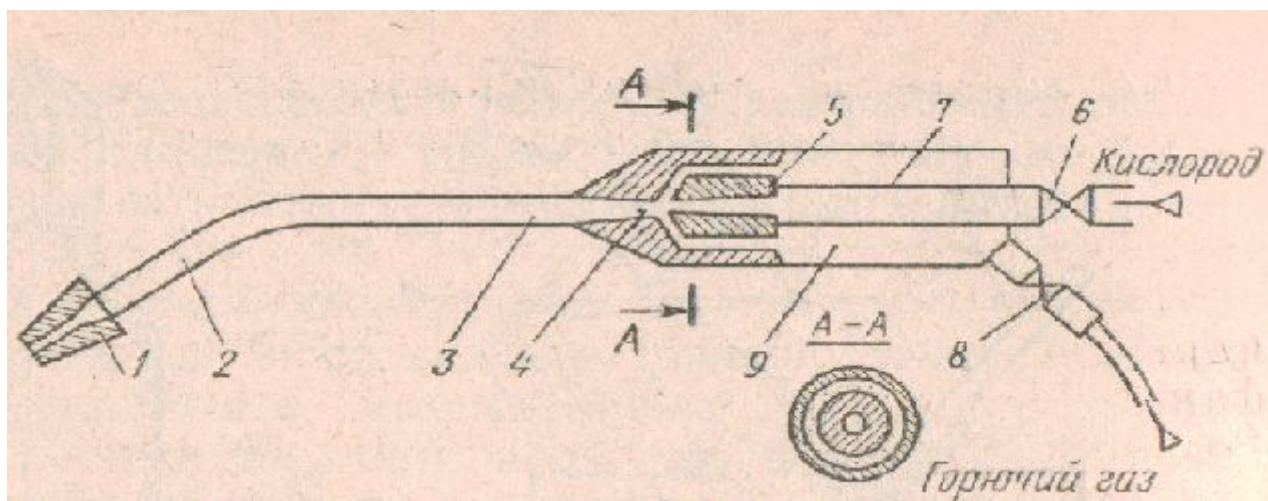
Газовая сварка
