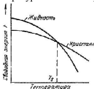
Рис.1. Изменение свободной энергии в зависимости от температуры
