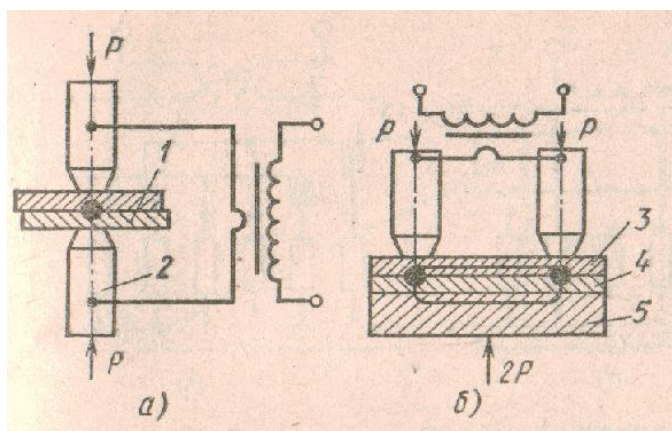
Точечная сварка
