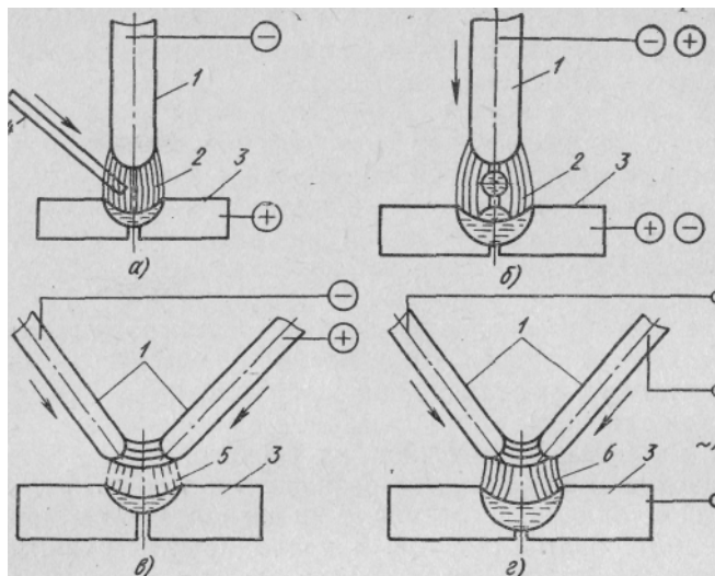
Электродуговая сварка
