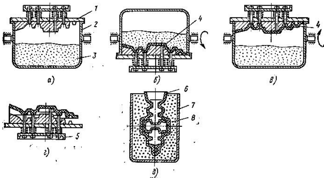
Литьё в оболочковые формы
