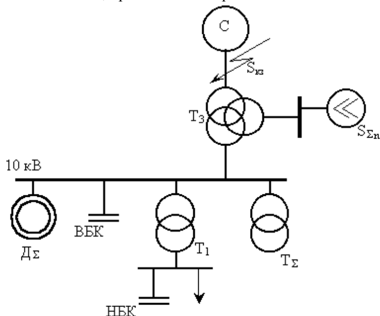
Рис. 1. Схема сети
