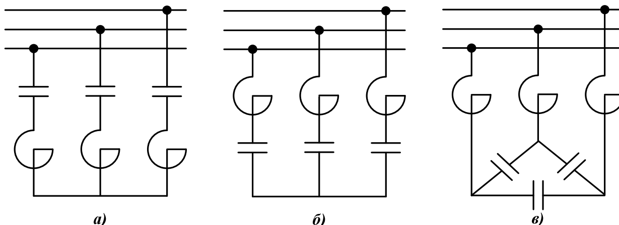
Рис.1. Упрощенные принципиальные схемы фильтров
