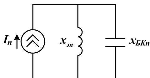
Рис.1. Эквивалентная схема замещения
