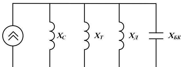
Схема замещения.
