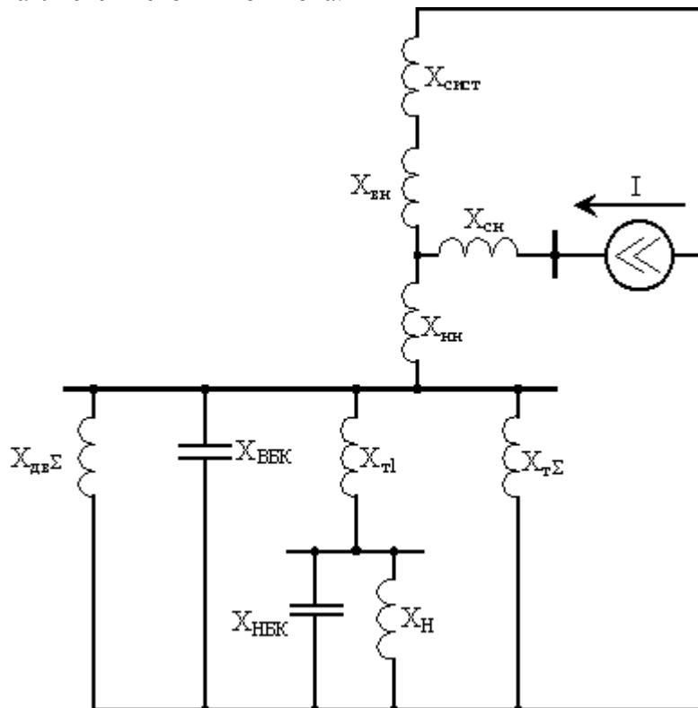
Рис. 2. Схема замещения
