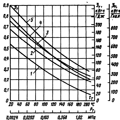
Рис.1. Удельная суммарная выработка электроэнергии на внешнем и внутреннем теплоснабжении.
