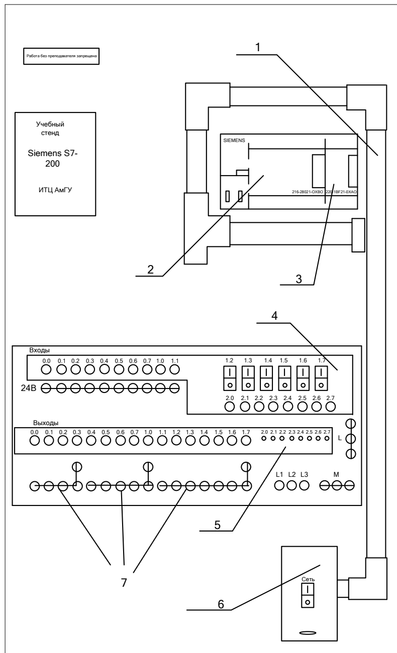
Рис. 4. Внешний вид стенда
