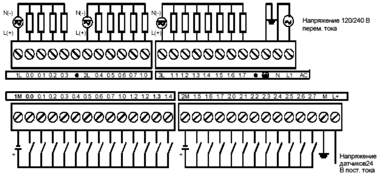
Рис. 5. Вариант схемы соединений CPU
