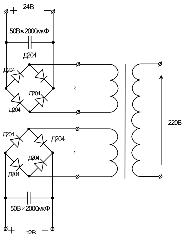
Рис. 3. Принципиальная электрическая схема питания
