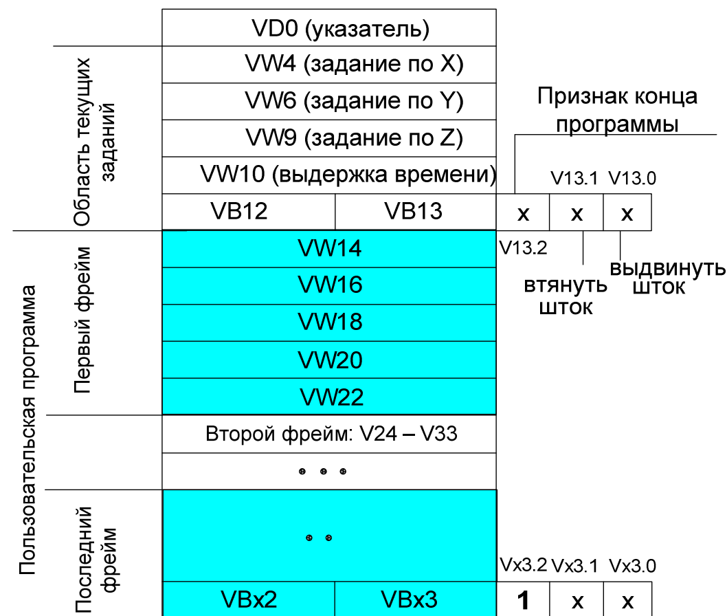
Рис. 12. Использование памяти области V
