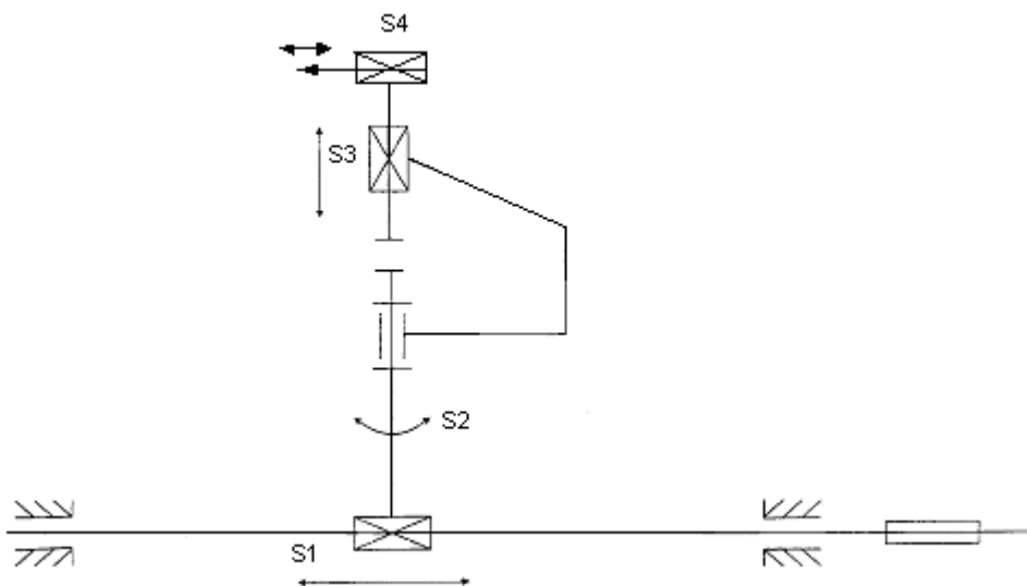
Рис. 1. Кинематическая схема
