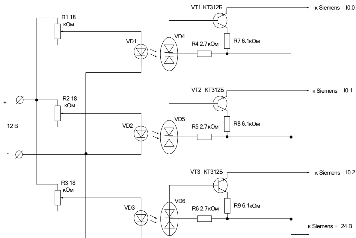
Рис. 6. Схема системы измерения положения рабочего органа
