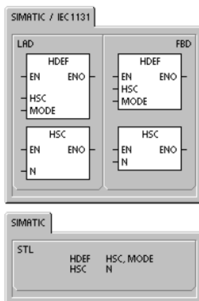
Рис. 3. Команды управления скоростными счетчиками
