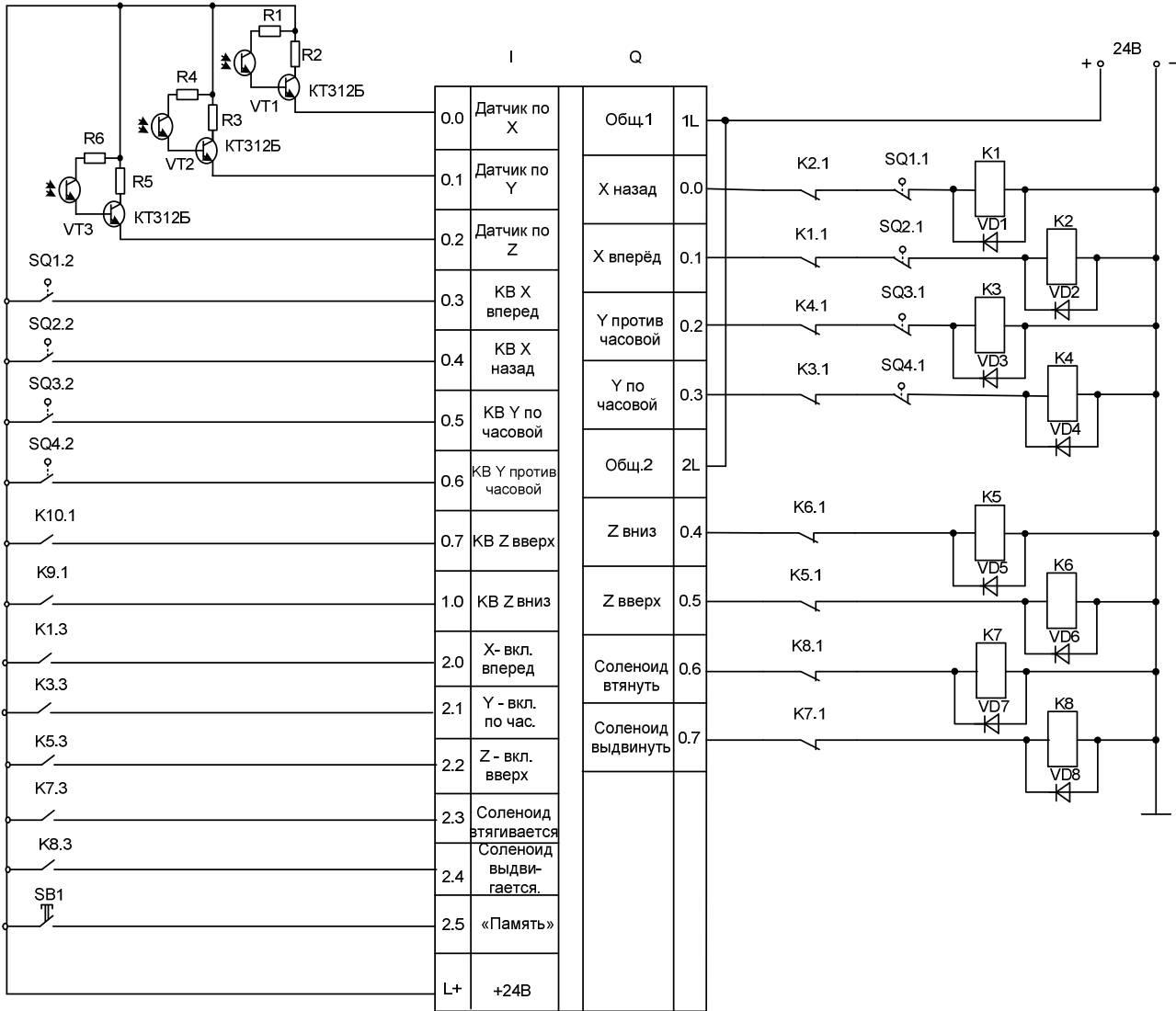
Рис. 7. Рекомендуемая схема подключения робота манипулятора к станку
