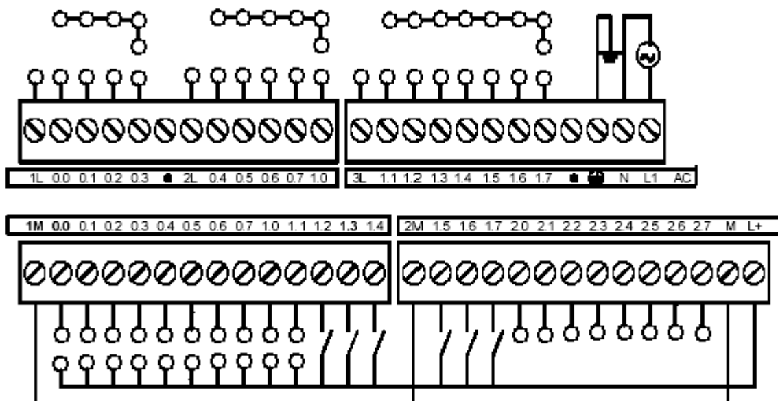
Рис. 6. Разводка внешних цепей CPU на стенде
