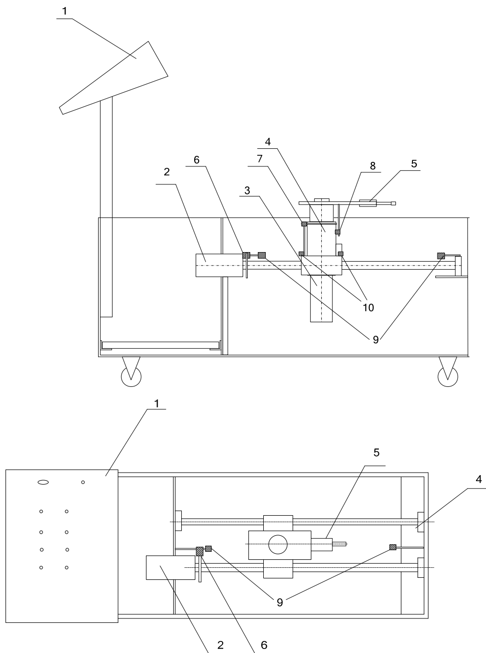
Рис. 2. Внешний вид робота-манипулятора
