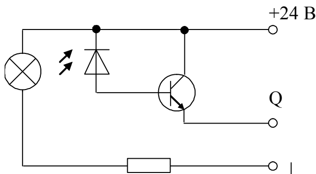
Рис. 2. Принципиальная схема датчика
