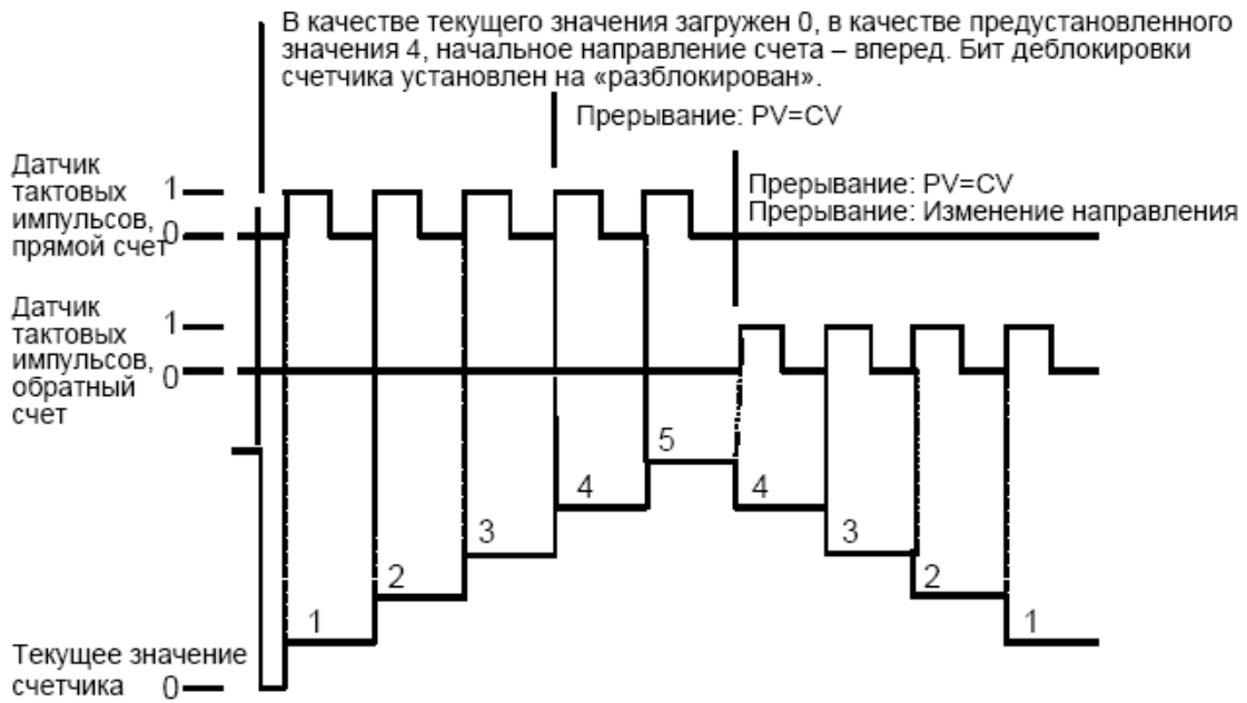
Рис. 6. Пример работы в режимах 6, 7 или 8
