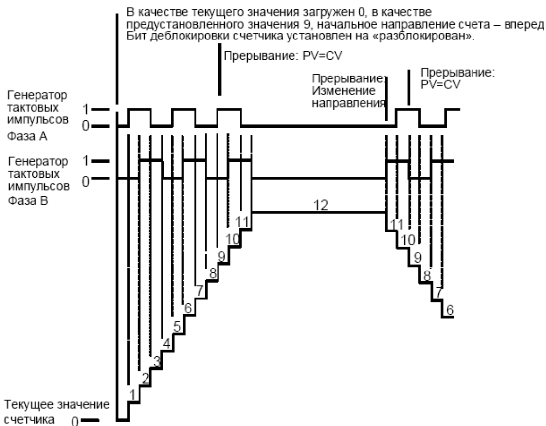
Рис. 8. Пример работы в режимах 9, 10 или 11 (квадратурный режим, четырехкратная скорость)
