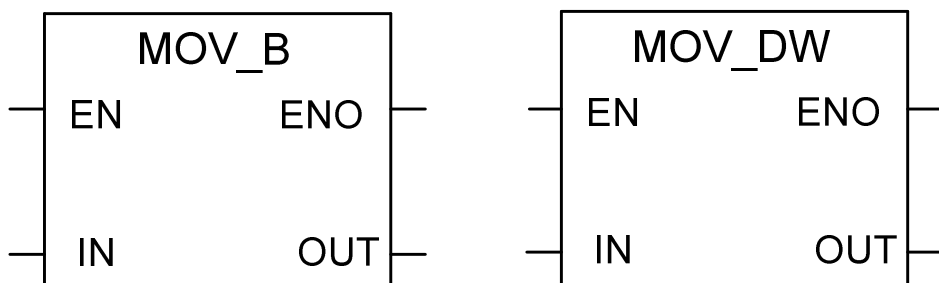
Рис. 11. Команда пересылки слова и двойного слова
