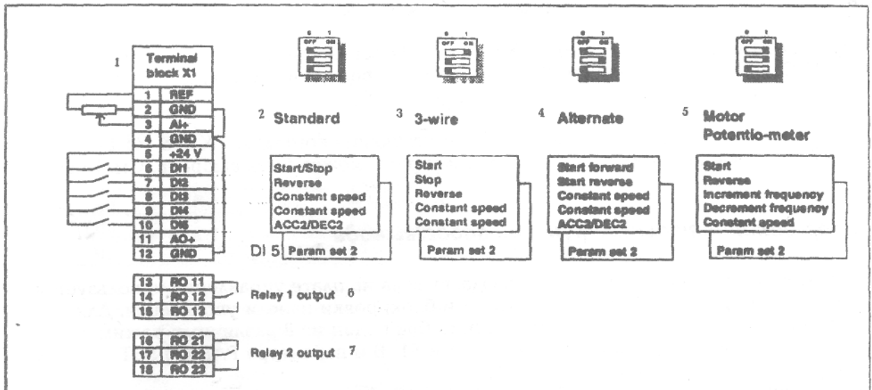
Рис. 2. Схема соединений цепей управления
