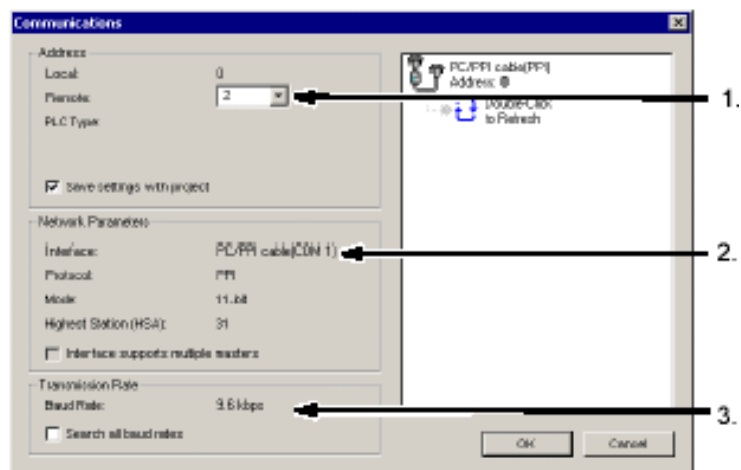
Рис. 2. Проверка параметров обмена данными
