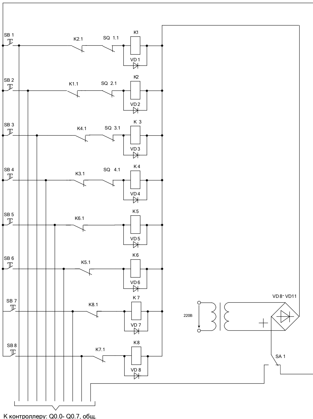
Рис.5. Схема цепей коммутации (ручное управление)
