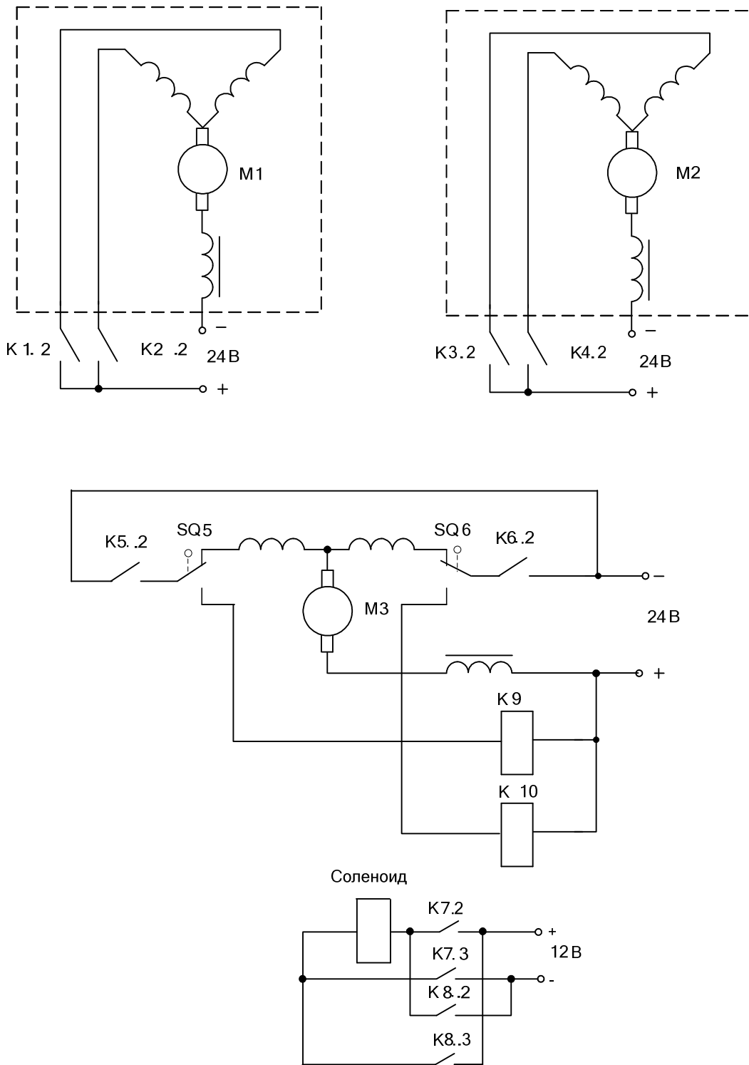
Рис. 4. Схема силовых цепей
