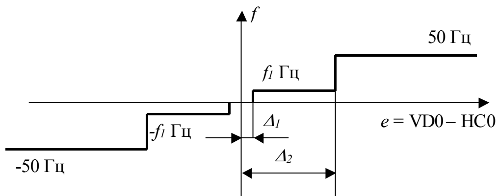
Рис. 1. Алгоритм регулирования угла поворота
