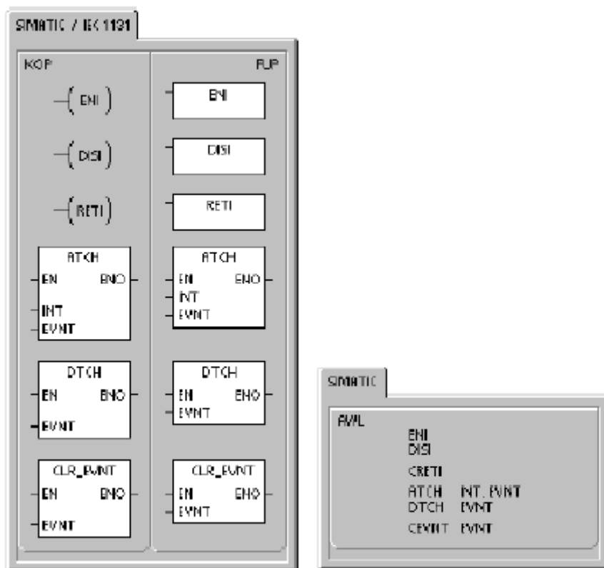
Рис. 10. Команды прерываний Siemens S7–200
