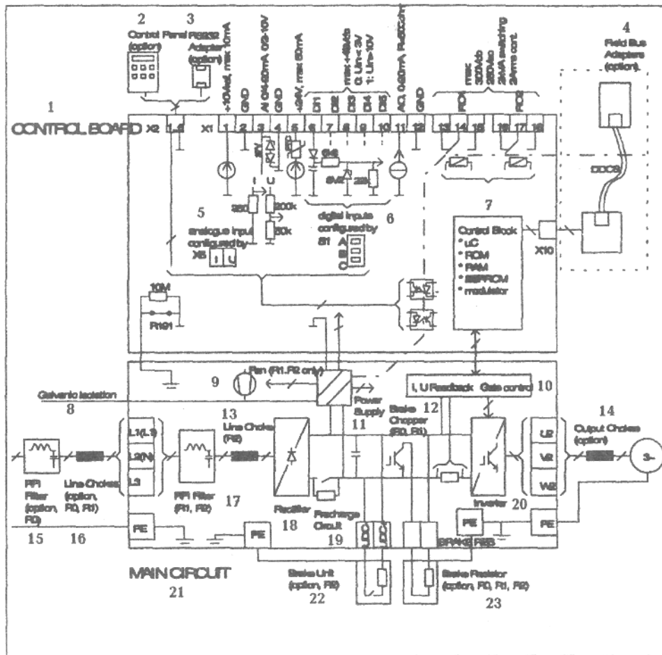
Рис 1. Блок-схема ACS 300.
