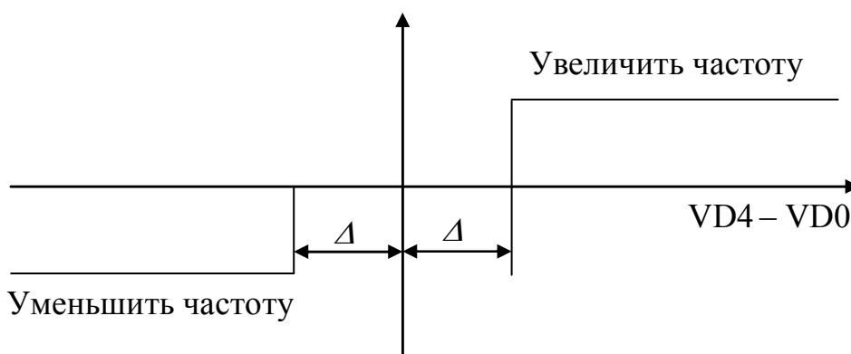
Рис. 2. Алгоритм регулирования частоты вращения
