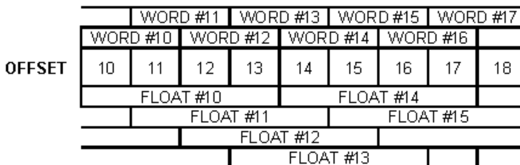
Рис. 6. Пересечения данных в S7 200
