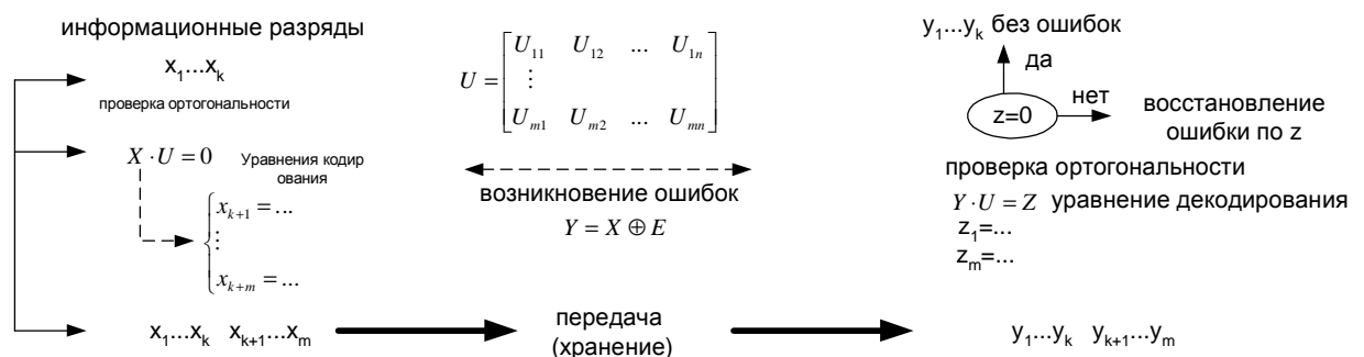
Рис.6.5 Схема кодирования и декодирования по Хеммингу
