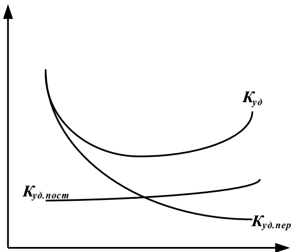
Рис. 15. Зависимость удельных капиталовложений от мощности оборудования электростанции
