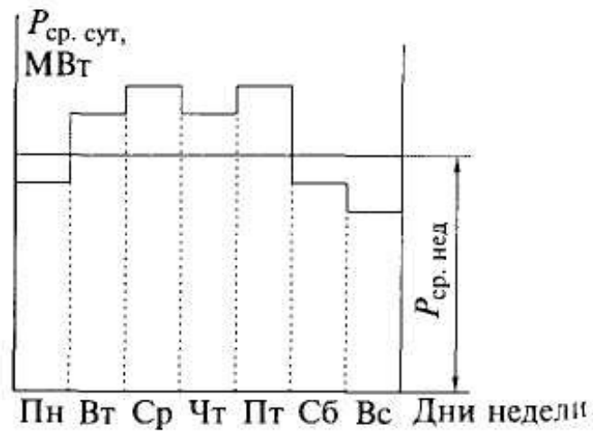
Рис. 3. График недельного электропотребления
