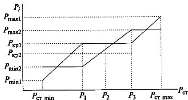
Рис. 33. Режимная карта машинного зала тепловой станции
