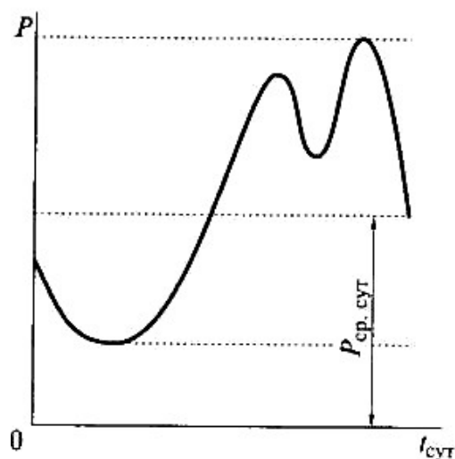
Рис .1. Суточный график нагрузки
