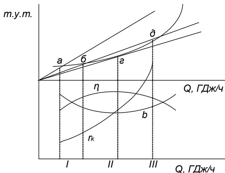
Рис. 21. Взаимосвязь между удельным расходом топлива, относительным приростом расхода топлива и КПД котла: I – зона сниженных нагрузок; II – зона средних нагрузок; III – зона повышенных нагрузок
