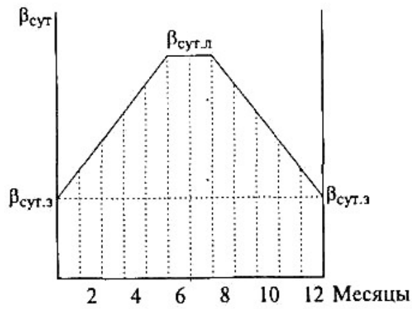
Рис. 4. Годовые графики нагрузки
