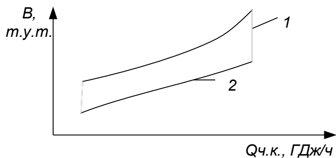
Рис 19. Расходная характеристика котла:
