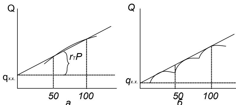
Рис. 23. Расходные характеристики паровых турбоагрегатов при замене криволинейных зависимостей прямолинейными: a – для одного турбоагрегата; б – для нескольких турбоагрегатов
