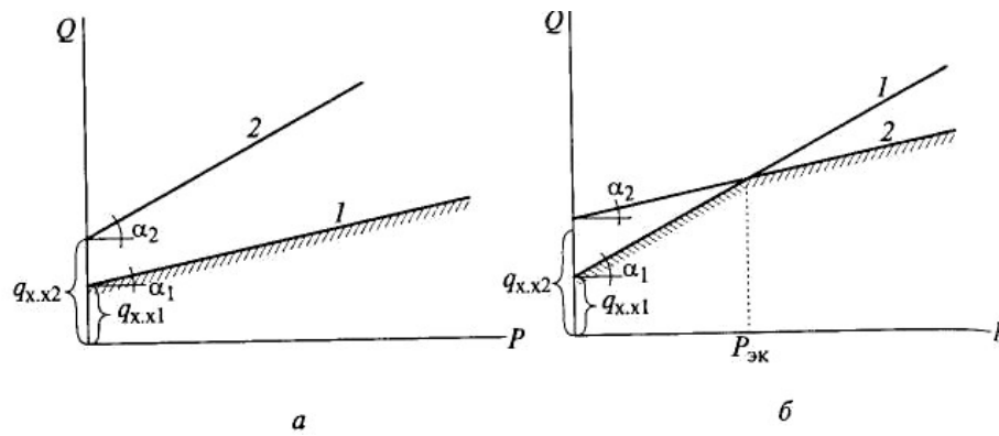
Рис. 31. Полное покрытие нагрузки ТЭС одним из агрегатов: а – нагрузка ТЭС полностью покрывается турбиной № 1; б – в зоне P < P_{эк} нагрузка ТЭС полностью покрывается турбиной № 1, в зоне P > P_{эк} – полностью турбиной № 2; 1, 2 – расходные характеристики турбин
