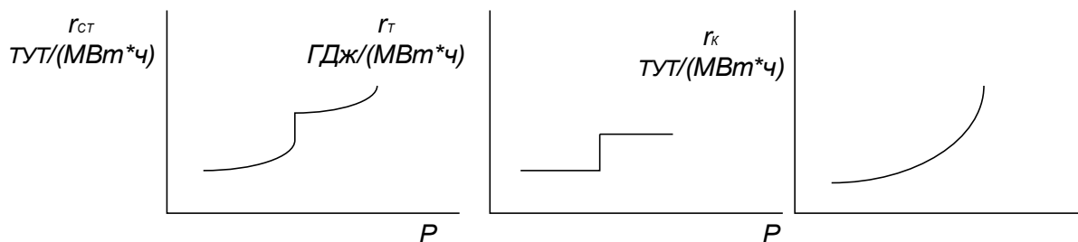
Рис. 30. Построение характеристики относительных приростов расхода топлива тепловой электростанцией: а – электростанции; б – турбоагрегата; в – котла
