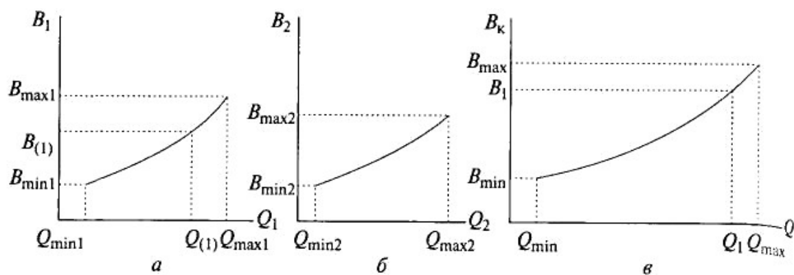
Рис. 29. Энергетические характеристики: а – первого котла; б – второго котла; в – котельной
