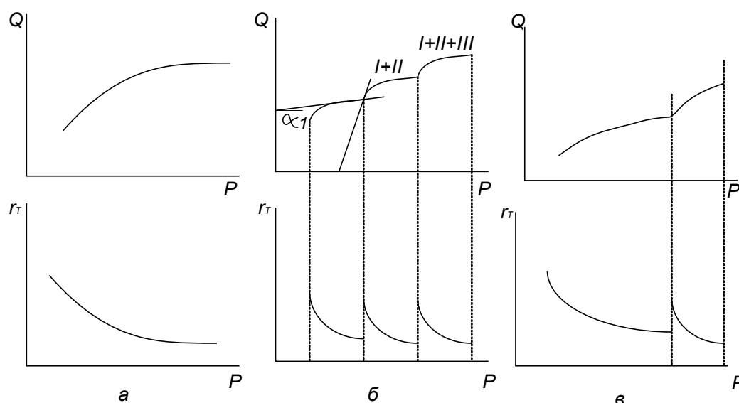
Рис. 22. Расходные характеристики паровых турбоагрегатов:
