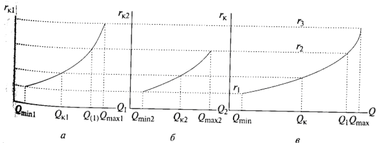
Рис. 28. Построение характеристики относительных приростов расхода топлива котельной: а – первого котла; б – второго котла; в – котельной
