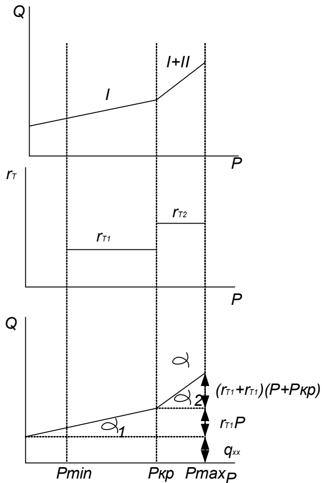
Рис. 24. Расходная характеристика паровых турбоагрегатов при обводном регулировании: I, II – клапаны
