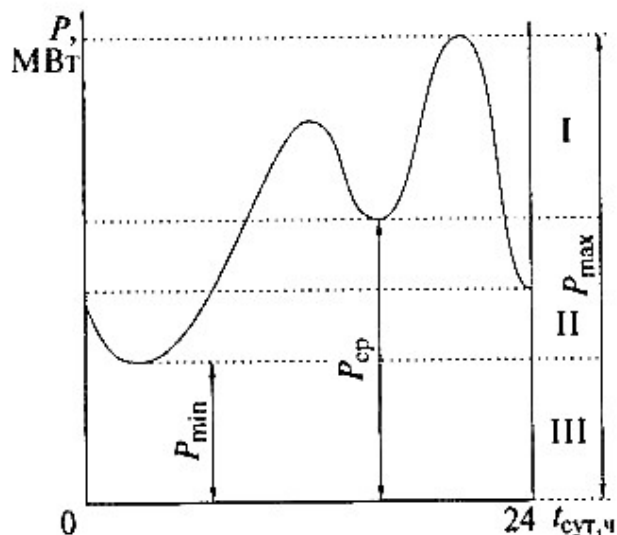
Рис. 2. Составляющие части суточного графика нагрузки: I, II, III – пиковая, полупиковая, базисная
