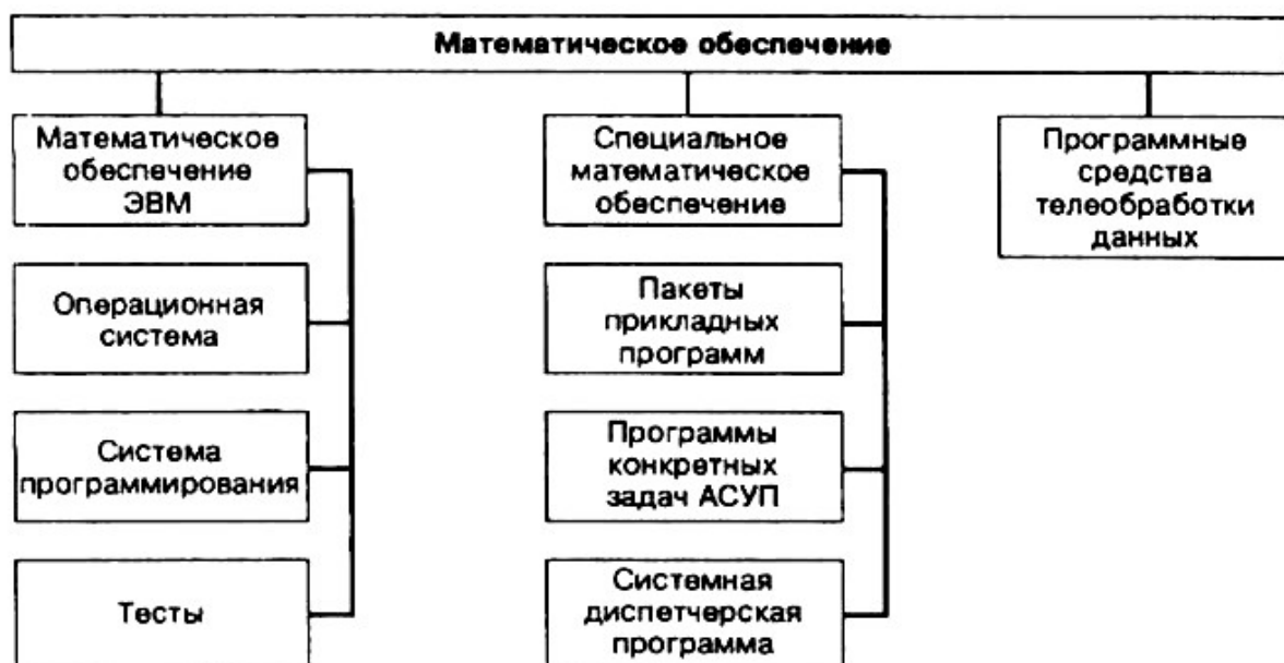
Рис. 38. Классификация математического обеспечения.
