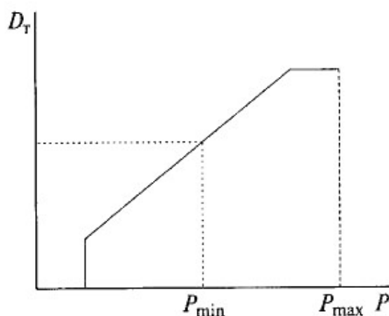
Рис. 25. Определение параметров (коэффициентов) расходной характеристики турбоагрегата на основе диаграммы режима
