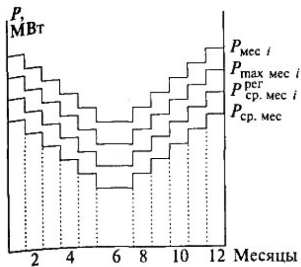
Рис. 5. Изменение значений коэффициента заполнения суточного графика
