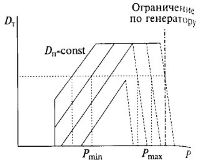
Рис. 26. Зависимость параметров расходной характеристики турбоагрегата от величины отборов пара
