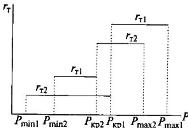
Рис. 32. Относительные приросты расхода тепла турбоагрегатами по зонам нагрузки
