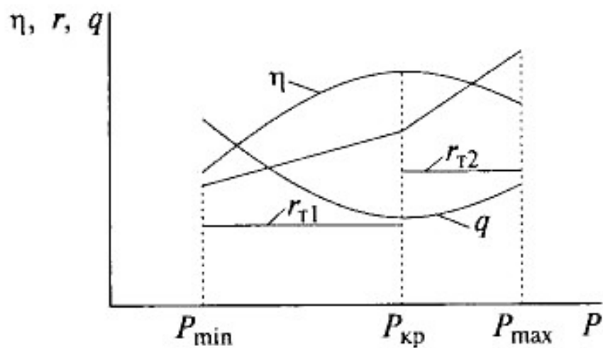
Рис. 27. Относительные показатели работы турбоагрегатов
