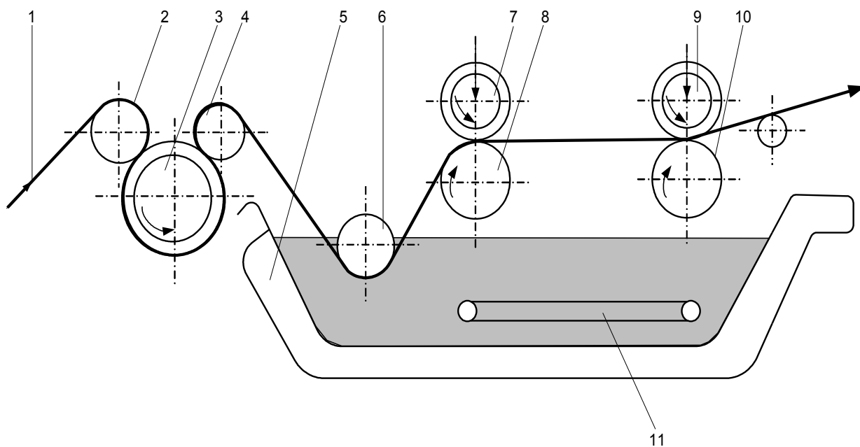
Рисунок 1 – Технологическая схема клеильного аппарата и отжимного устройства шлихтовальной машины
