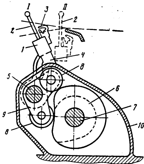
Рисунок 3 – Схема привода батанного механизма станка СТБ
