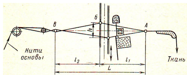
Рис. 169. Схема зева
