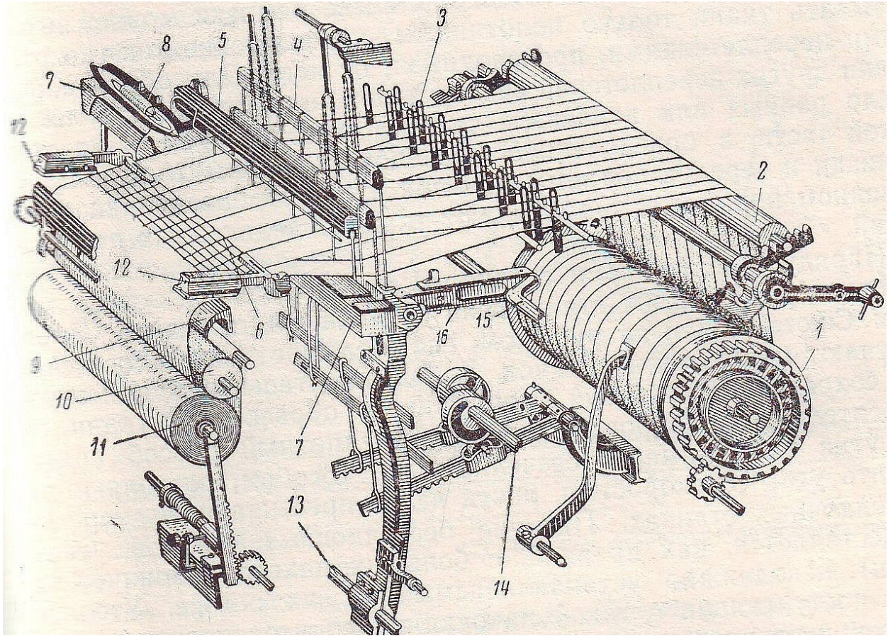
Рис.1.Ткацкий станок
