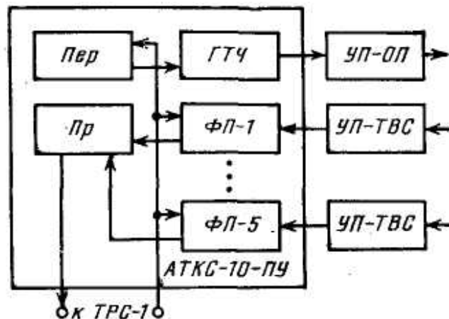
Рис. Функциональная схема АТКС-10 опорной подстанции ПУ
