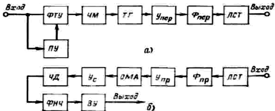
Рис. Функциональные схемы: а – модема передачи; б – модема приема
