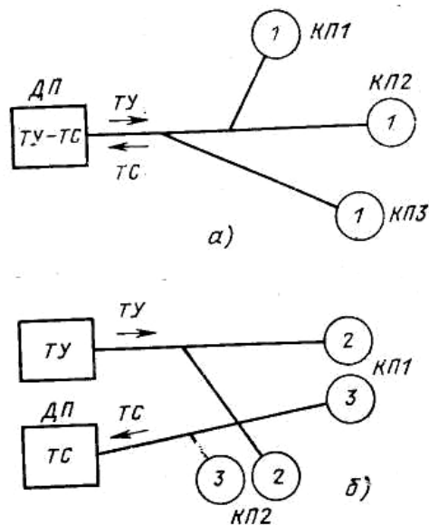
Рис. Многообъектные системы ТУ — ТС:
