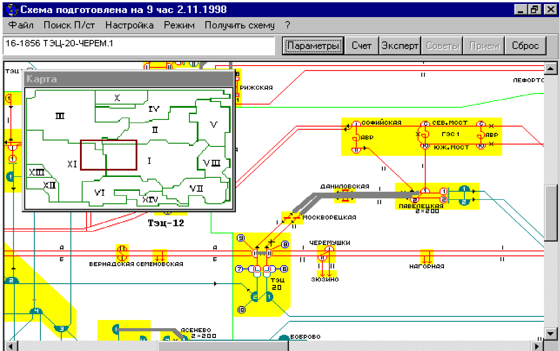
Рис. 5. Детальная схема «Тренэнерго»
