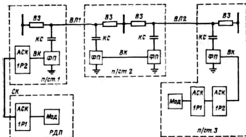
Рис. Функциональная схема сложного канала связи по ВЛ
