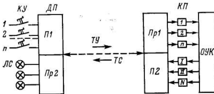
Рис. Структурная схема устройства ТУ — ТС:
