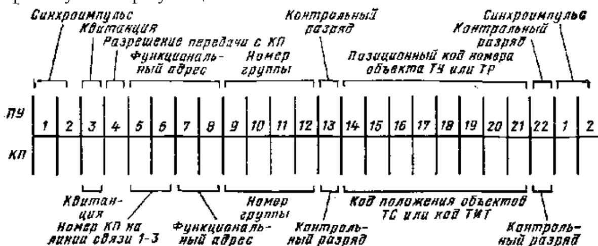
Рис. Диаграмма использования тактов распределителя в устройстве ТМ-320
