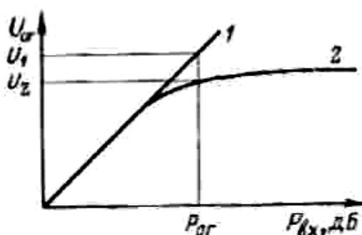
Рис. Амплитудная характеристика тракта приема модема
