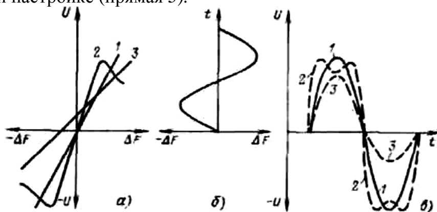
Рис. Частотные характеристики дискриминатора
