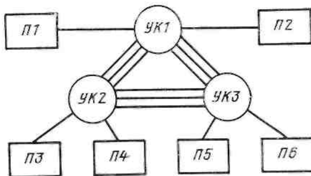
Рис. Функциональная схема автоматически коммутируемой сети передачи данных:
