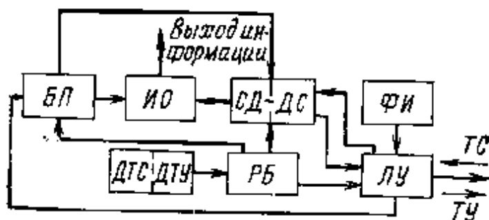
Рис. Структурная схема устройства ТМ-800
