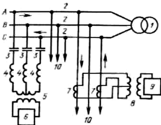
Рис. Схема подключения модема к ВЛ по схеме «фаза — фаза»
