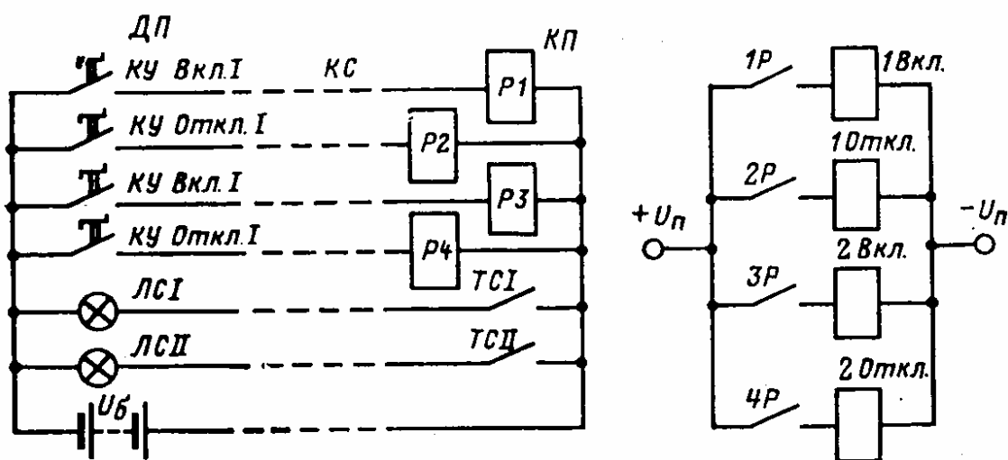
Рис. Принцип построения системы ТУ—ТС ближнего действия
