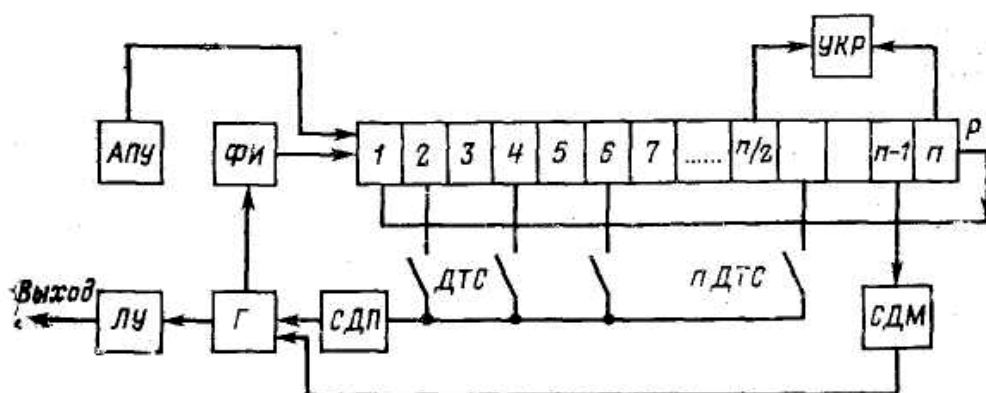
Рис. Структурная схема передатчика ТС устройства ВРТФ-1
