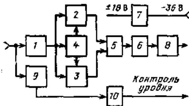
Рис. Функциональная схема линейного узла приема устройства МКТ-3
