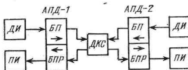
Рис. Функциональная схема СПД с некоммутируемым каналом связи
