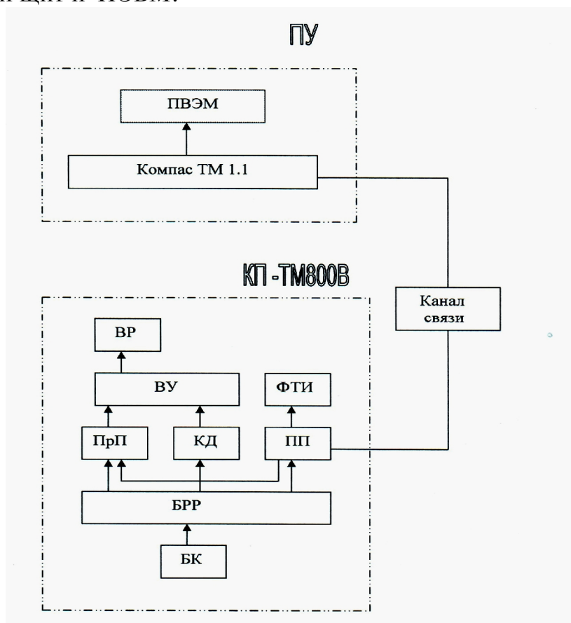
Рис. 1 – Конструктивное исполнение комплекта Компас ТМ 1. 1
