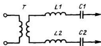
Рис. Схема устройства присоединения УП-КП-К.
