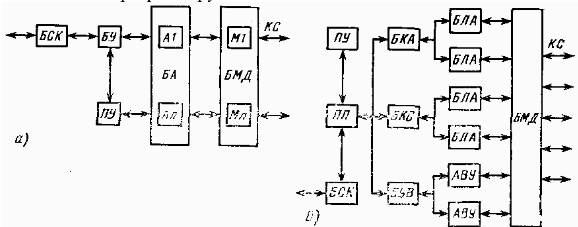
Рис. Функциональные схемы мультиплексора передачи данных: а - аппаратное исполнение; б - программированное исполнение
