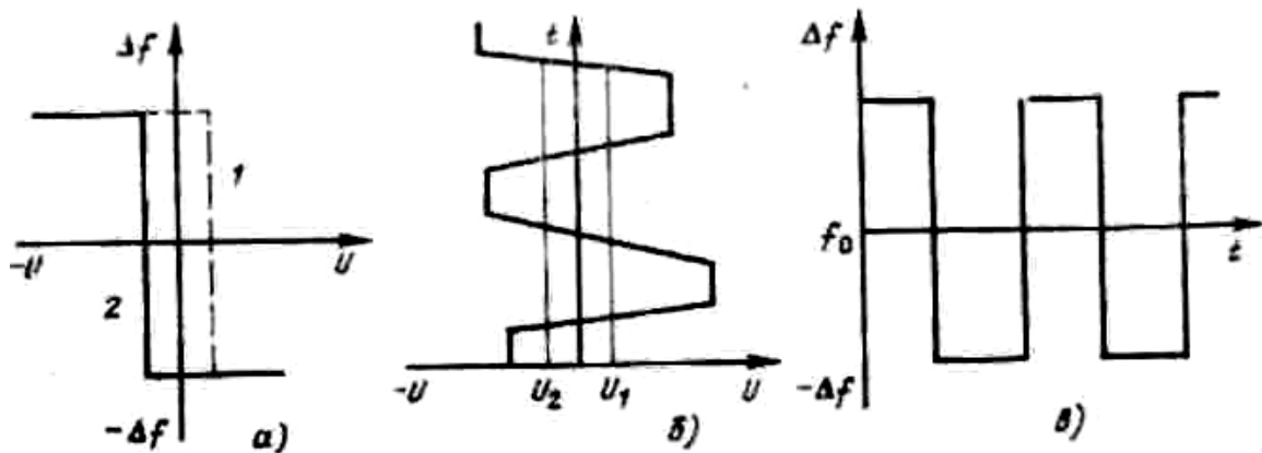
Рис. Модуляционная характеристика (а) и осциллограмма первичного сигнала на входе модема передачи (б) и форма ЧМ сигнала на входе модема (в)
