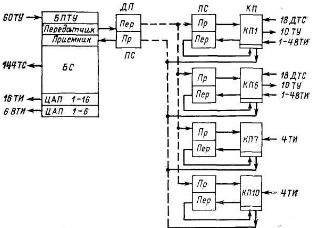
Рис. Структурная схема устройства КУСТ-Б
