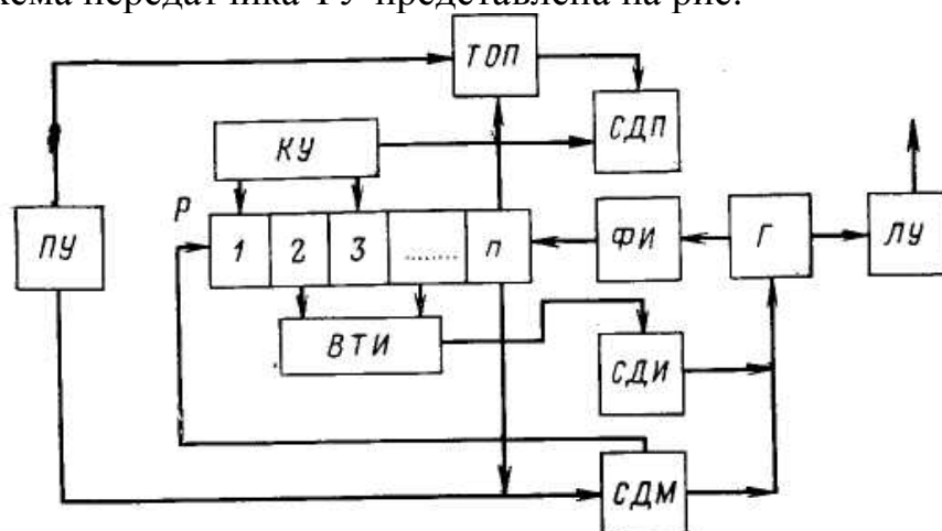
Рис. Структурная схема передатчика ТУ устройства ВРТФ-1
