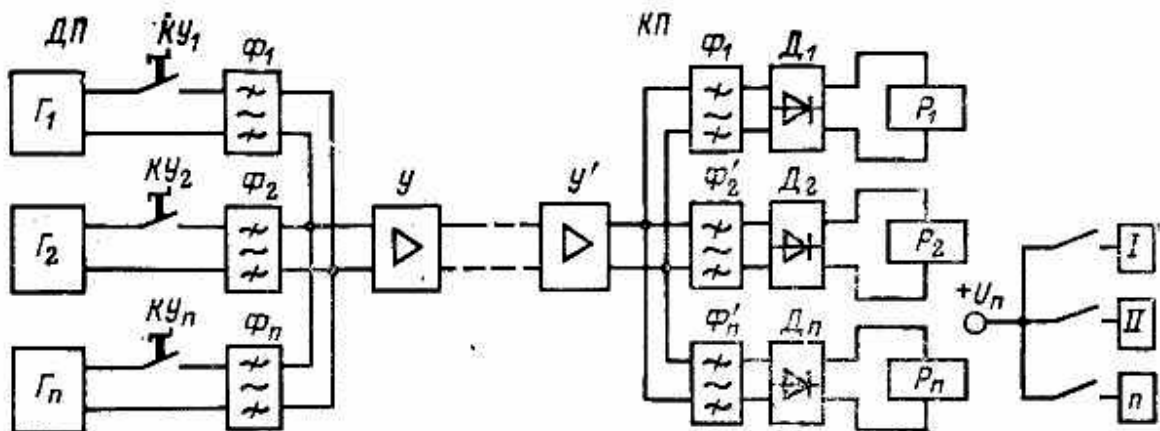
Рис. Частотное устройство ТУ — ТС
