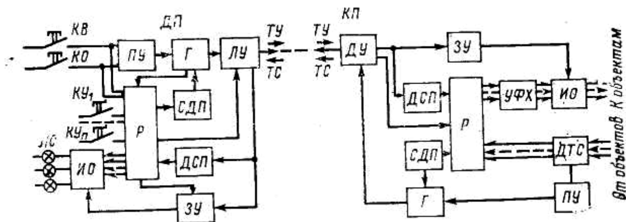
Рис. 8.6. Времязасоряющее контактное устройство ТУ — ТС
