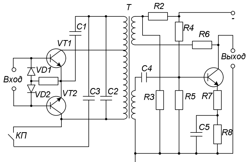
Рис. Принципиальная схема частотного модулятора и генератора тональной частоты
