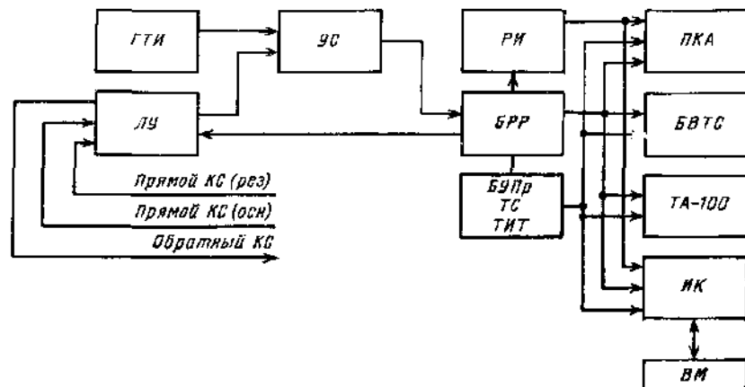
Рис. Структурная схема устройства КП комплекса ТМ-512
