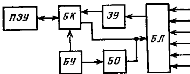
Рис. Функциональная схема узла коммутации сообщений
