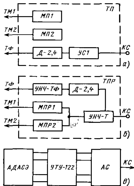
Рис. Функциональные схемы аппаратуры УТУ-122:
