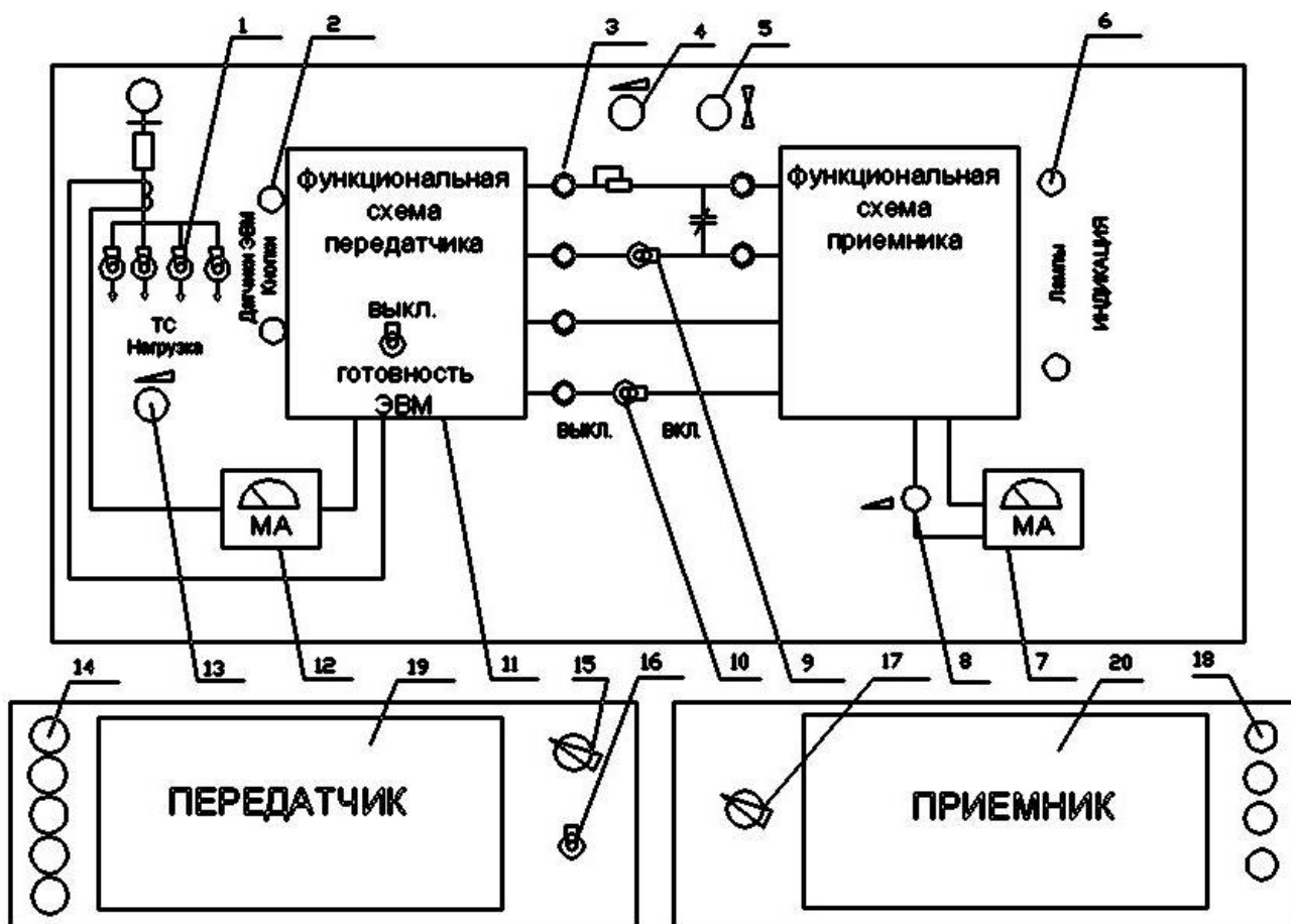
Рис. 2. Вид лабораторной установки
