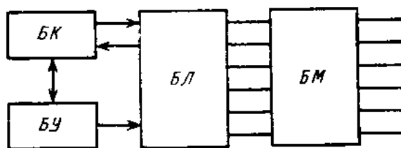
Рис. Функциональная схема узла коммутации каналов
