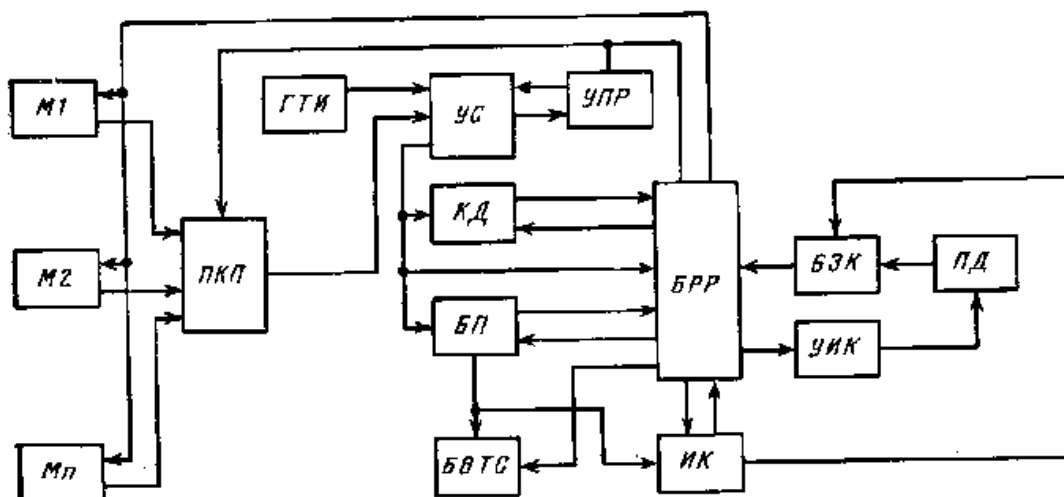
Рис. Структурная схема устройства ПУ телекомплекса ТМ-120
