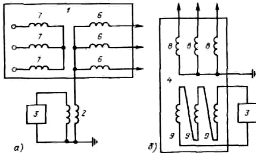
Рис. Схемы подключения модема к ВЛ по схеме «три фазы — земля»
