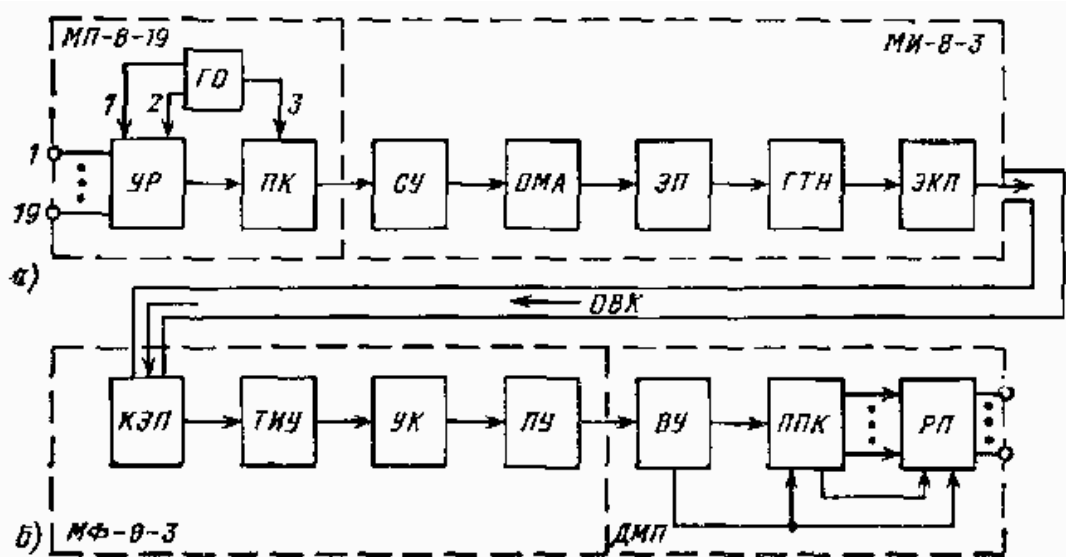
Рис. Система оптоволоконной передачи «Электроника МС4101»
