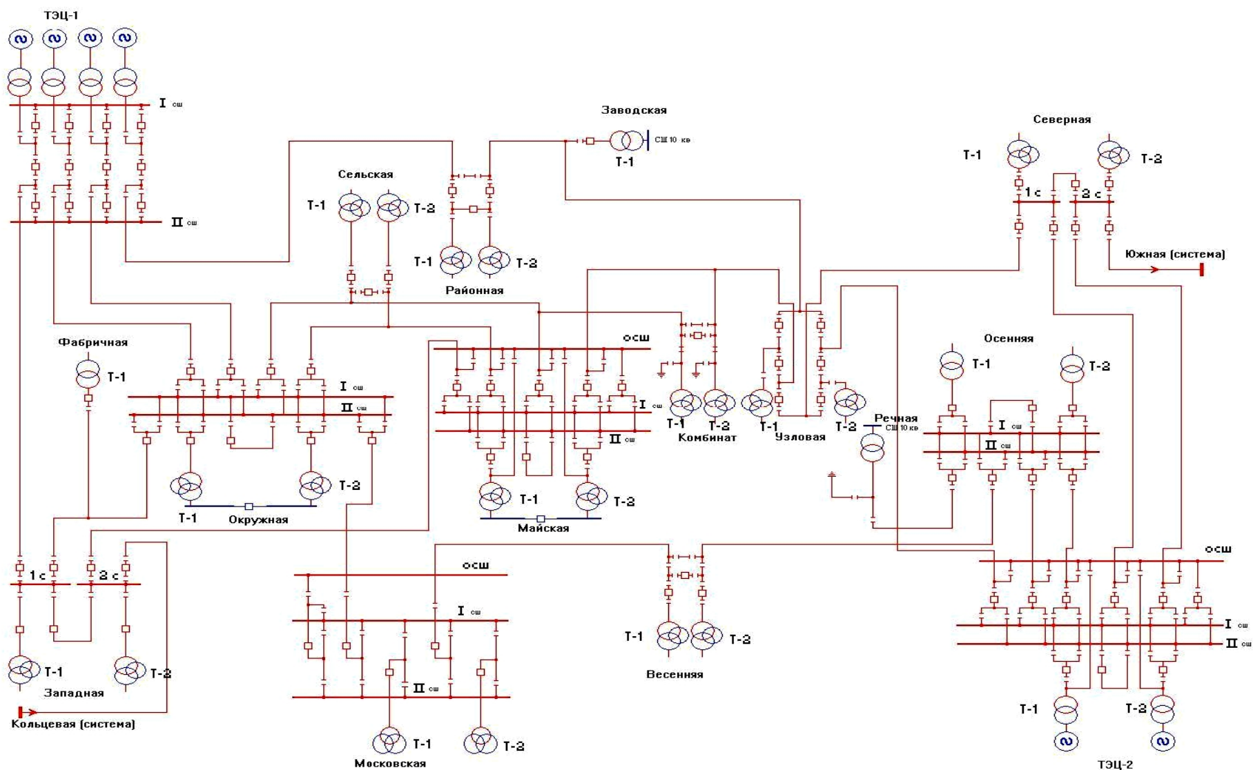
Рис. 4. Исходная электрическая схема «Тренэнерго»
