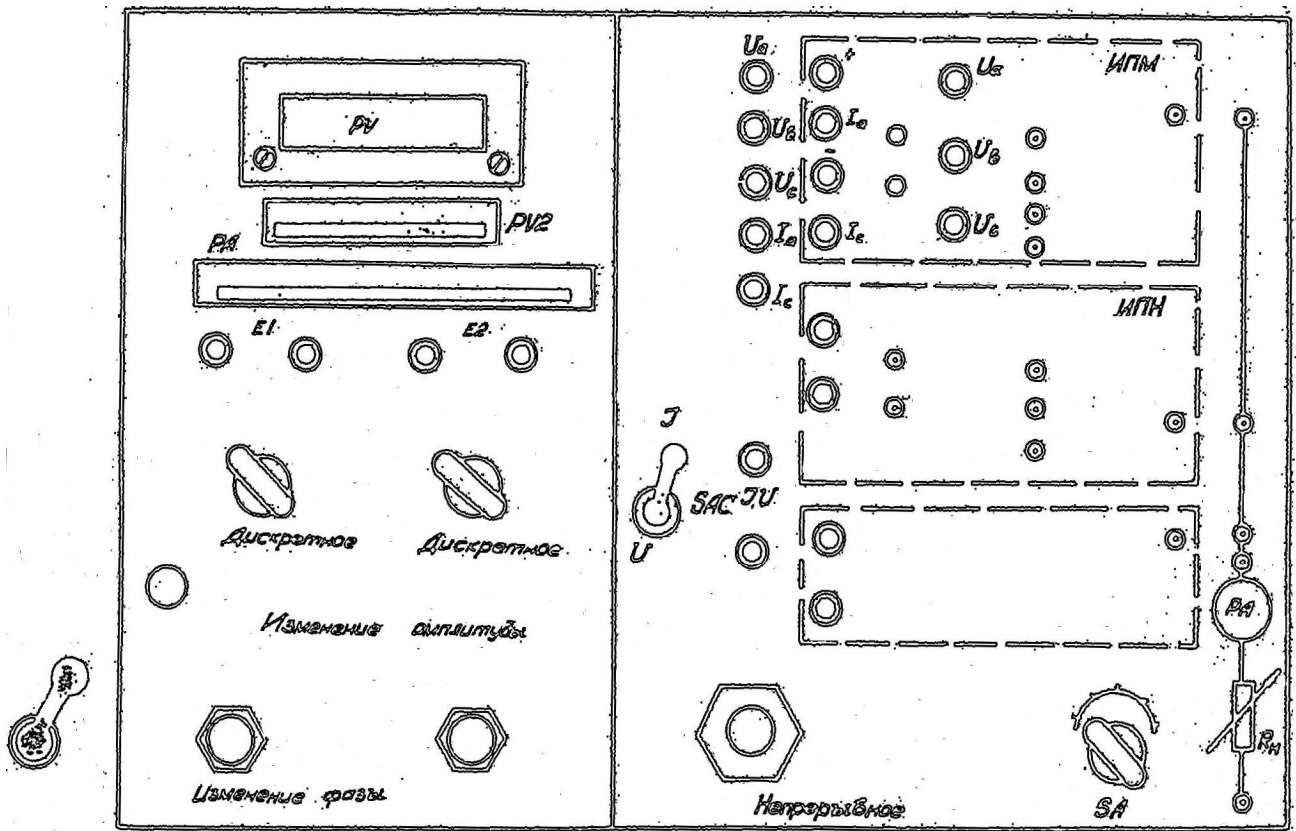
Рис. 3. Схема установки
