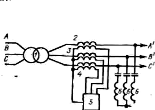
Рис. Схема подключения модема на КП по схеме «три фазы»
