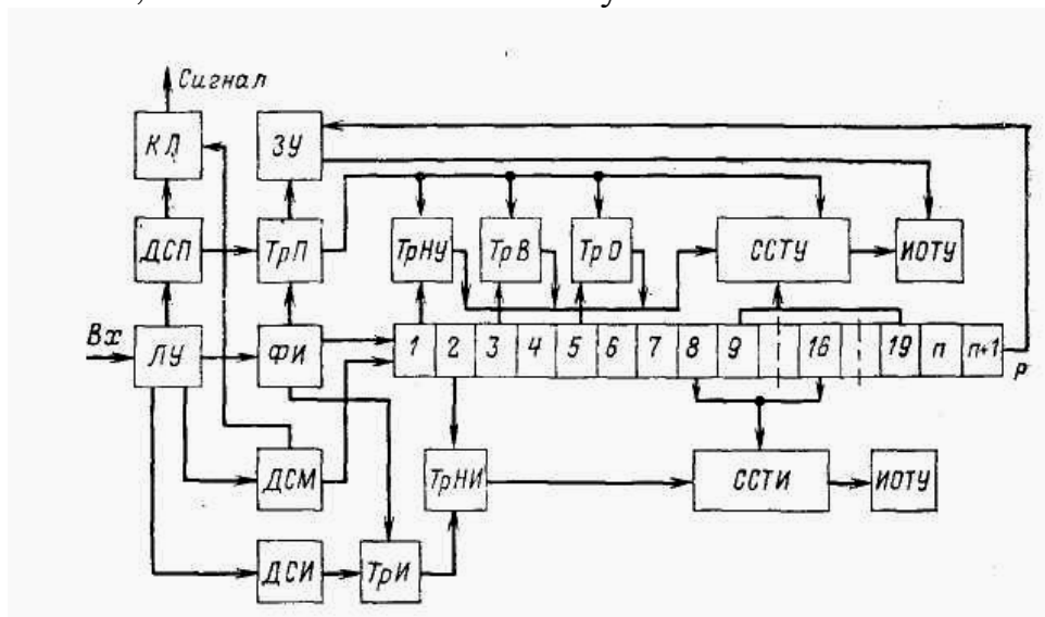
Рис. Структурная схема приемника ТУ устройства ВРТФ-1
