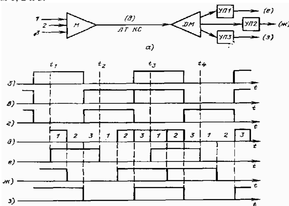
Рис. Метод мультиплексорной передачи
