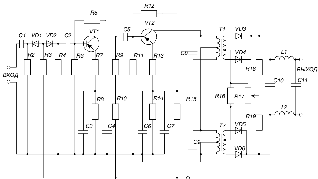
Рис. Принципиальная схема ограничителя максимальных амплитуд и частотного детектора
