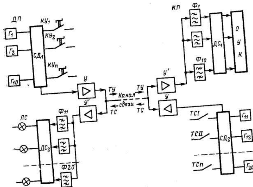
Рис. Частотно-комбинационное устройство ТУ — ТС
