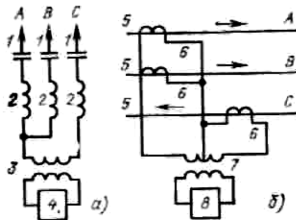
Рис. Схема подключения модема к ВЛ по схеме «две фазы - фаза»
