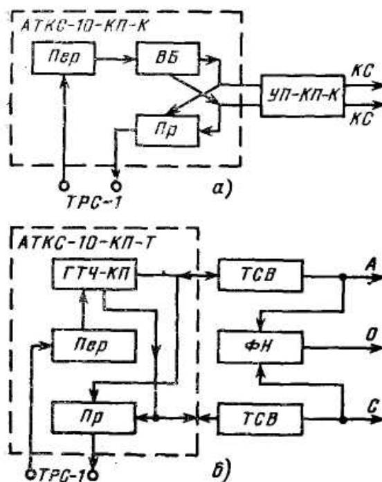
Рис. Функциональные схемы АТКС-10-КП
