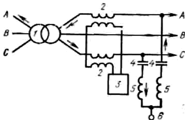
Рис. Схема подключения модема на КП по схеме «фаза- фаза»
