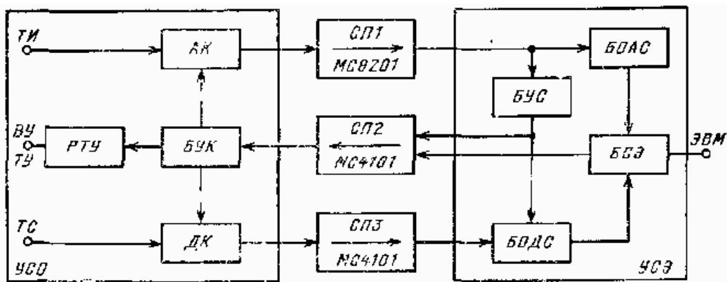
Рис. Структурная схема устройства телемеханики с элементами оптоволоконной техники
