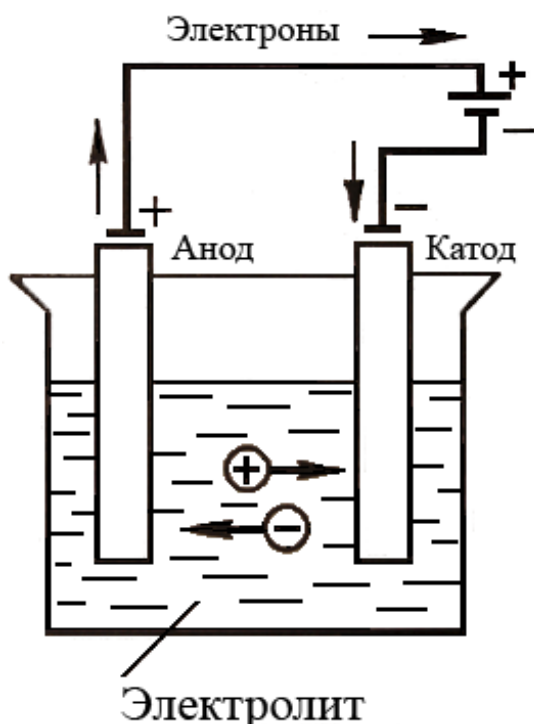
Рис. 19. Схема электролизера
