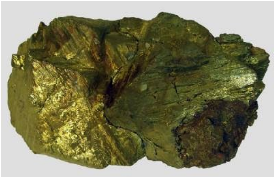
Рис. 7. Халькопирит
