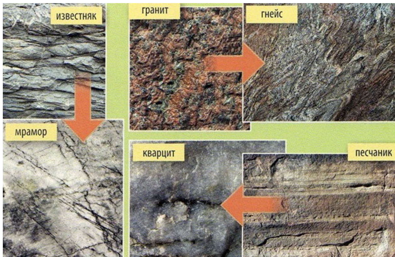
Рис. 58. Метаморфизм горных пород
