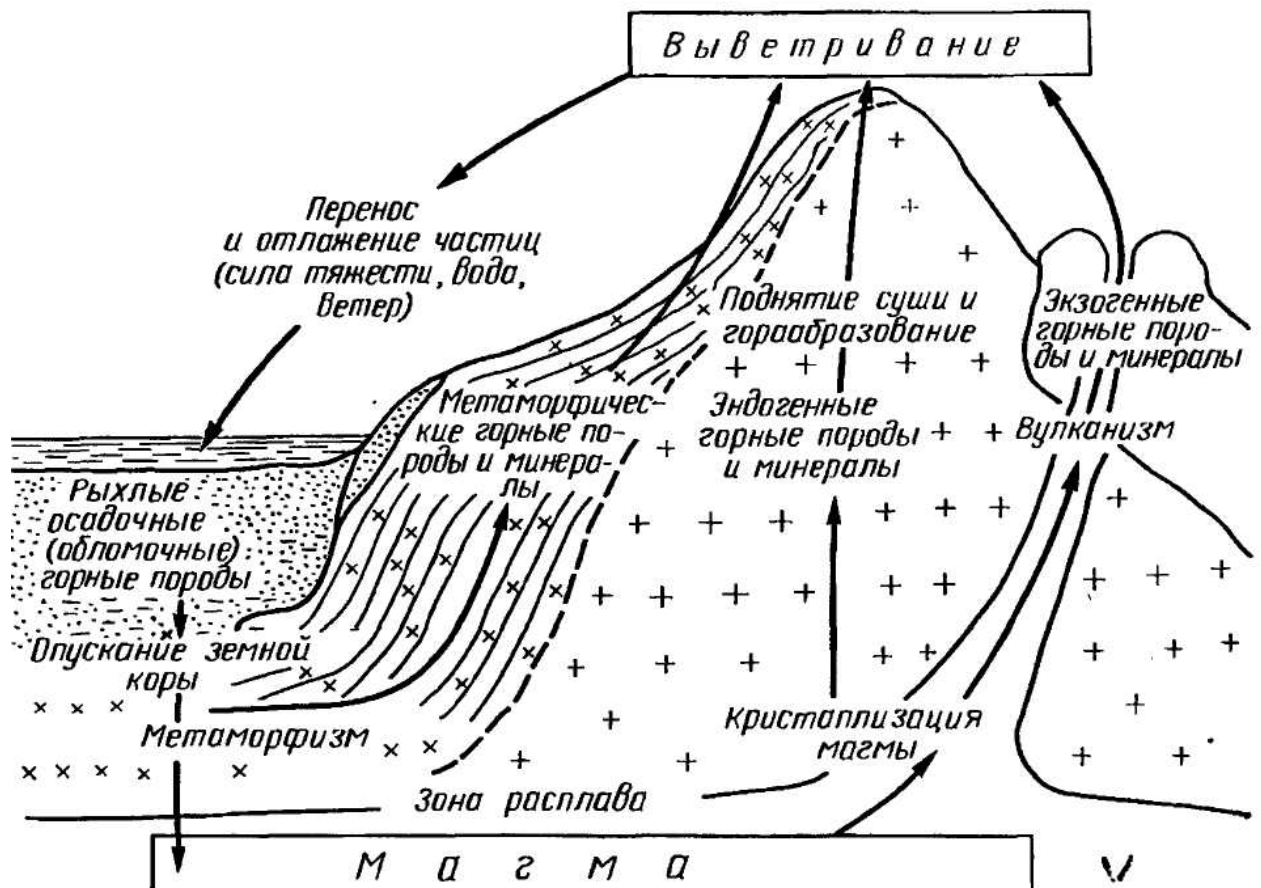
Рис. 21. Происхождение горных пород
