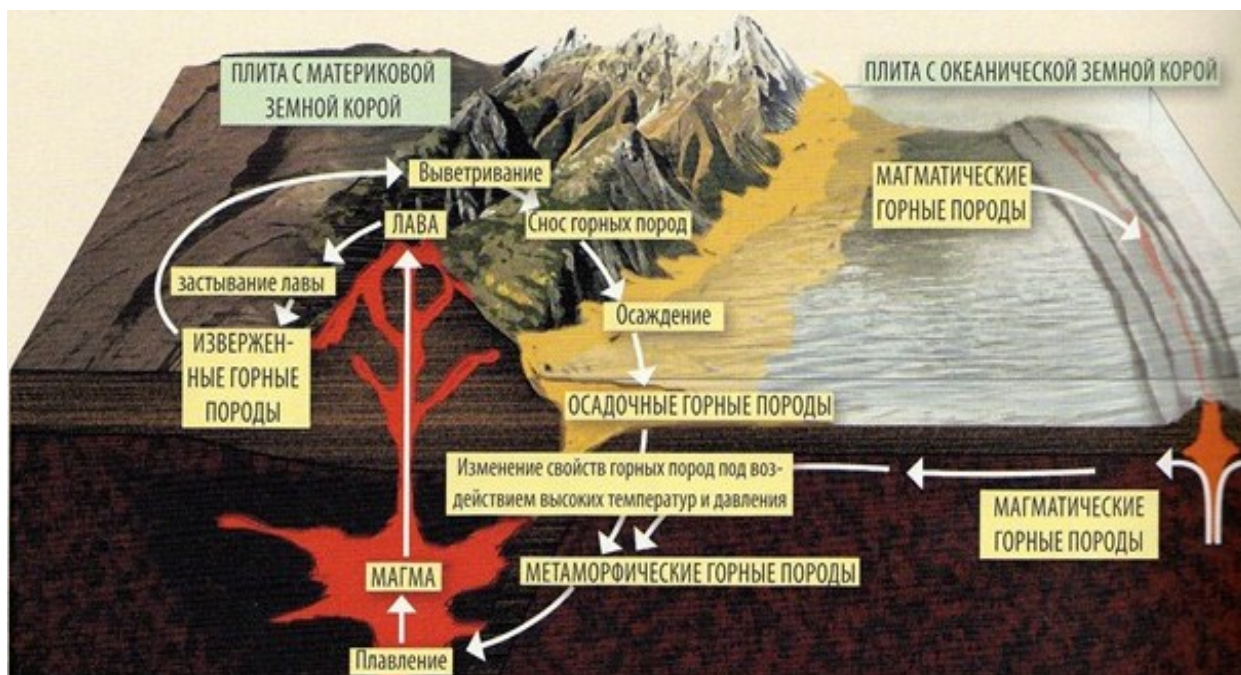
Рис. 23. Схема процесса круговорота горных пород
