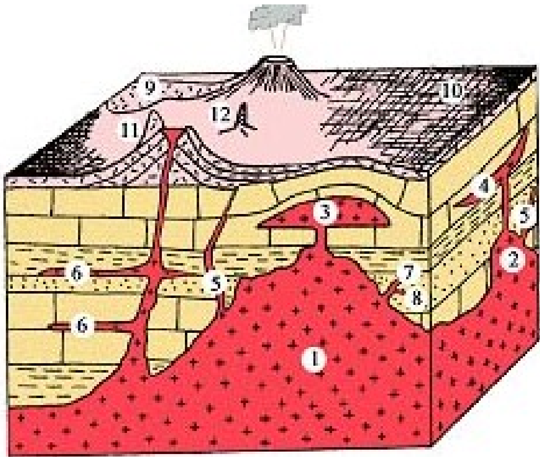
Рис. 31. Формы залегания магматических тел
