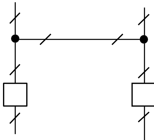
Рисунок 9 – 4Н - Два блока с выключателями и неавтоматической перемычкой со стороны линий
