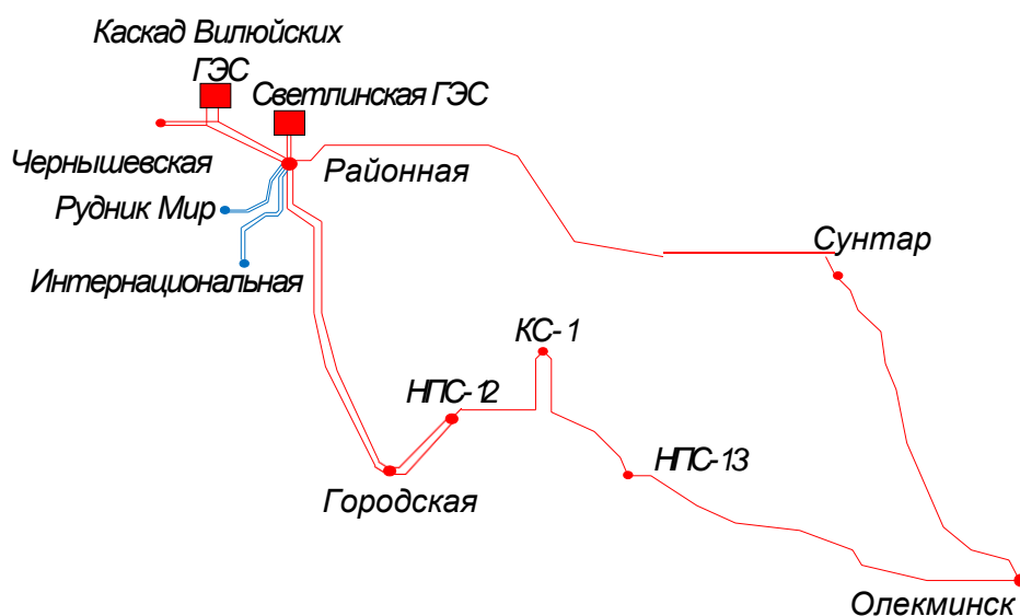
Рисунок 1 – Карта-схема рассматриваемого участка сети
