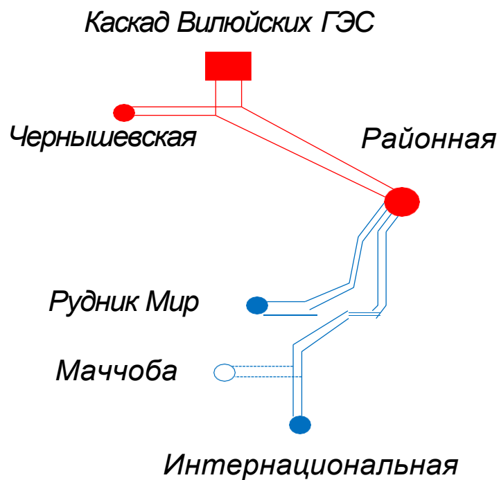
Рисунок 7 – Схема подключения № 1
