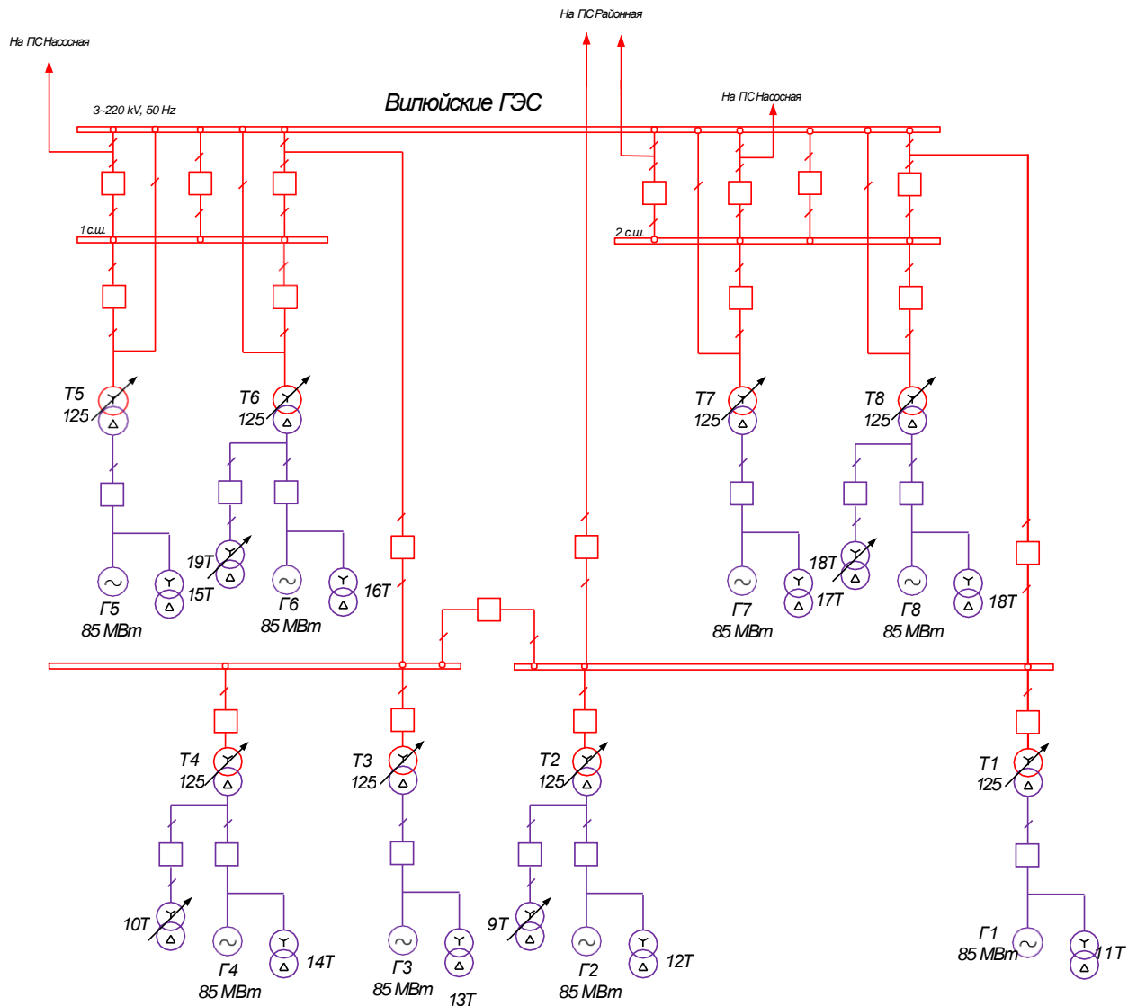
Рисунок 2 – Схема ОРУ Виллюйской ГЭС
