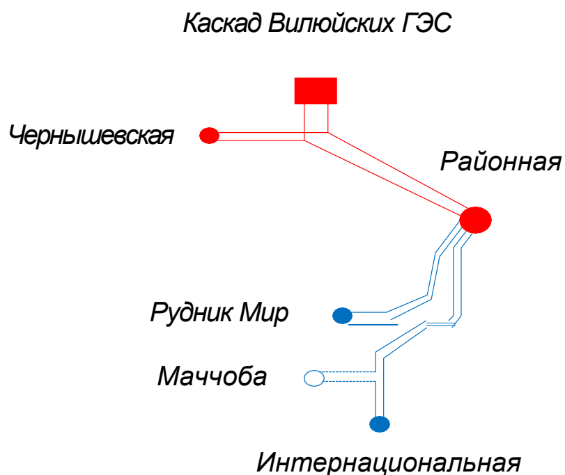
Рисунок 8 – Схема подключения № 2
