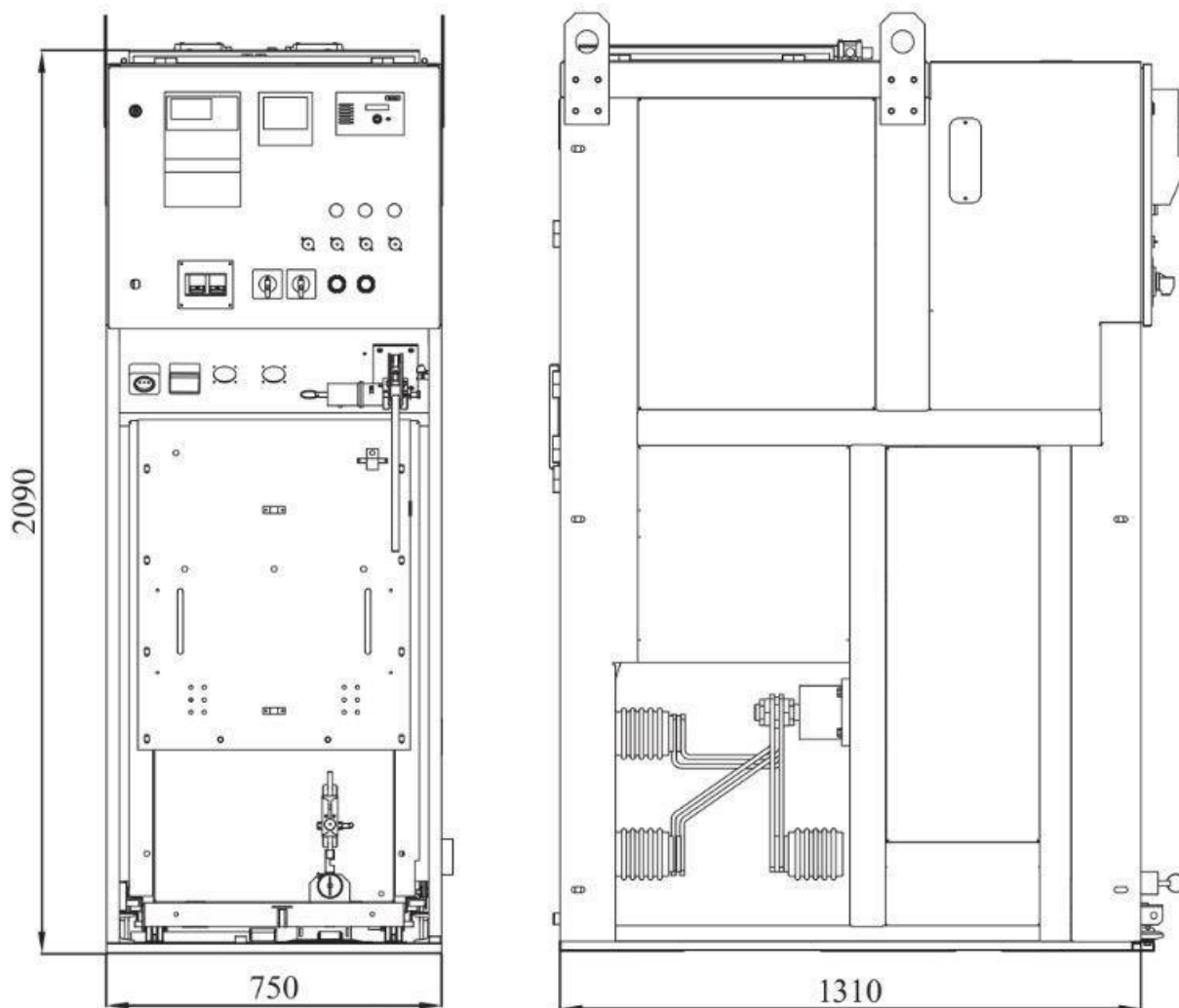
Рисунок 15 – КРУ К-104
