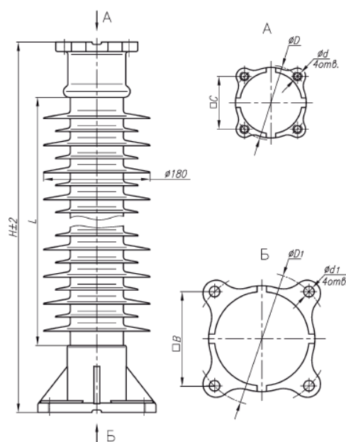
Рисунок 18 – Опорный изолятор ОСК 10-110-А-2 УХЛ1
