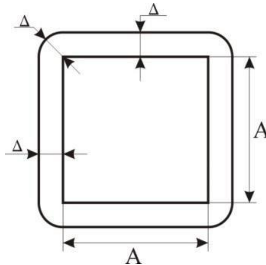
Рисунок 22 – К расчету площади земельных участков отводимых в постоянное пользование под стальные свободстоящие опоры ВЛЭП
