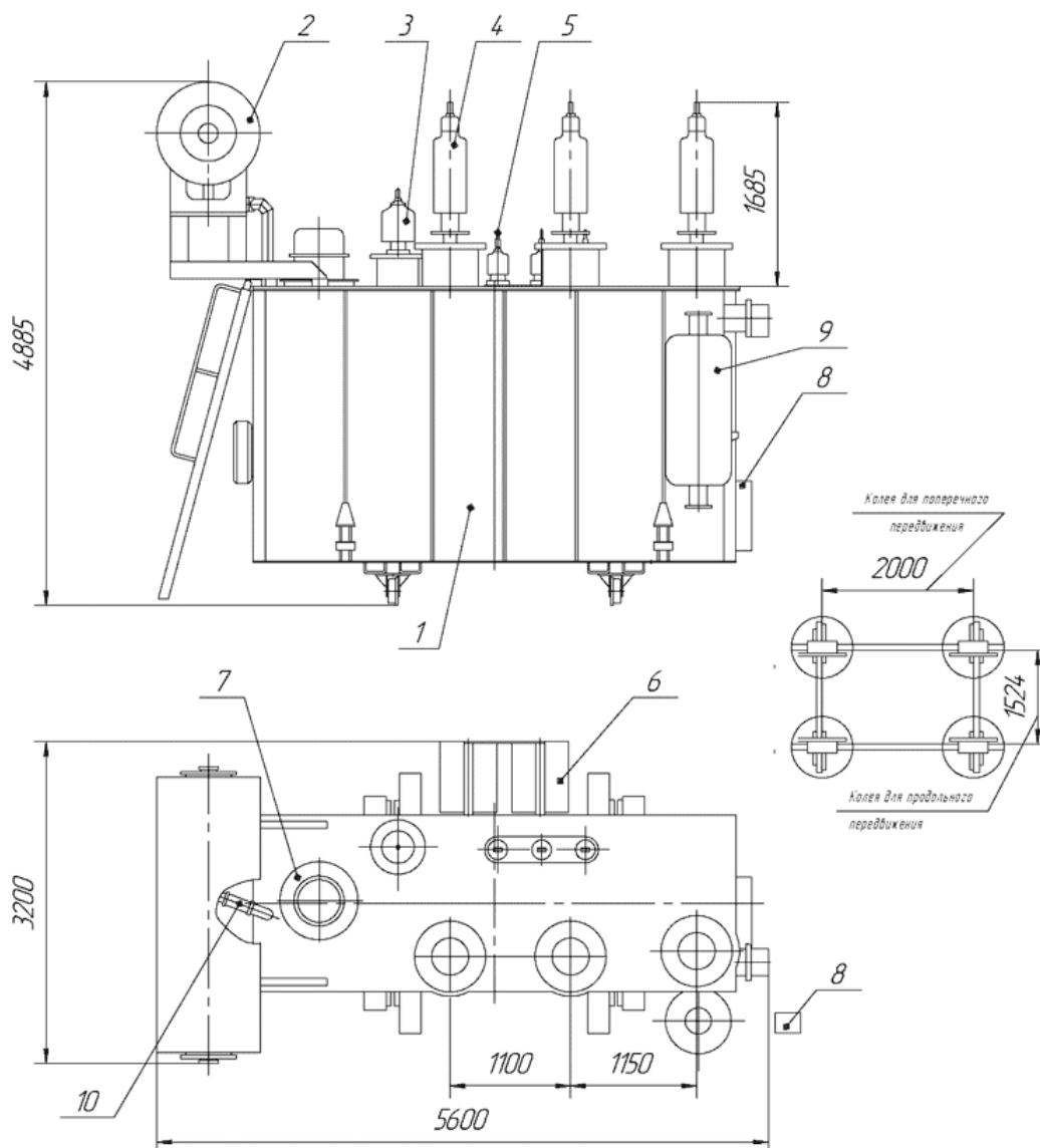
Рисунок 10 – Силовой трансформатор ТДН-10000/110
