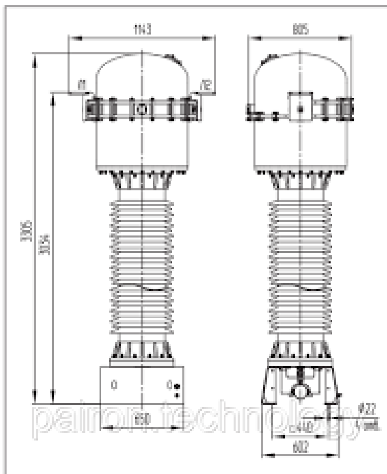
Рисунок 16 – Трансформатор тока ТОГФ-110-УХЛ1
