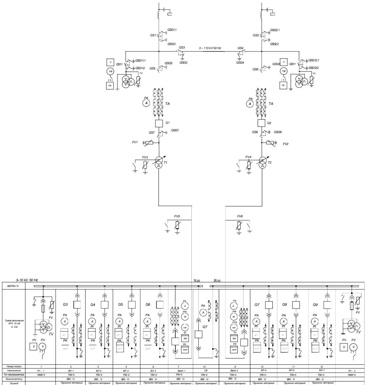
Рисунок 20 – Однолинейная схема ПС Маччоба
