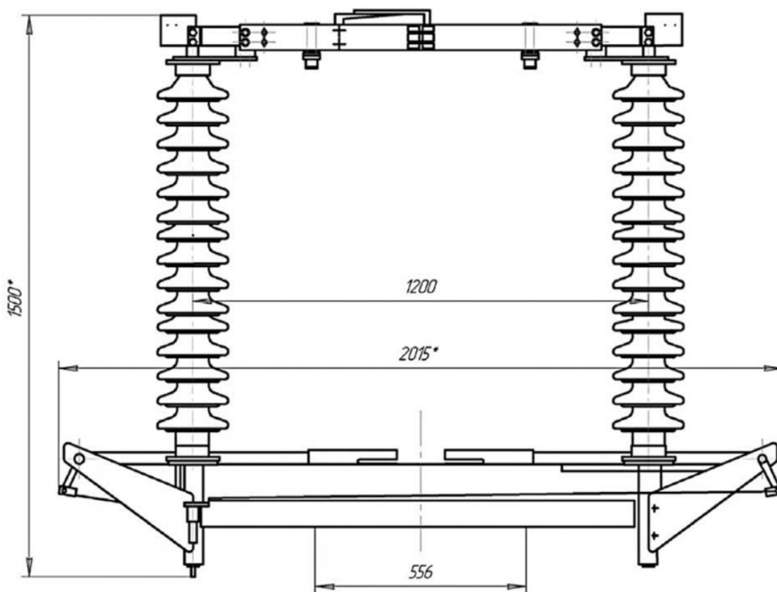
Рисунок 14 – Разъединитель РДЗ-110/1000 НУХЛ1
