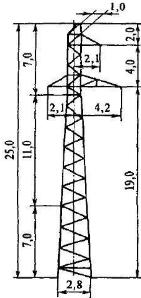
Рисунок 23 – Опора П-110-3
