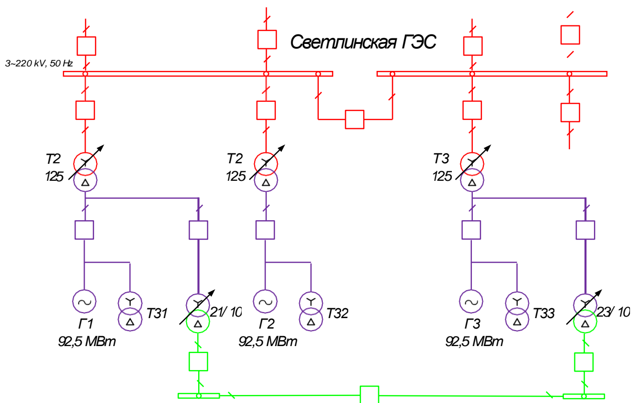
Рисунок 3 – Схема ОРУ Светлинской ГЭС
