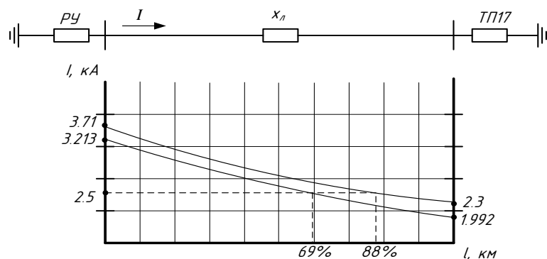
Рисунок 11 - График спадаания токов трехфазного КЗ по линии
