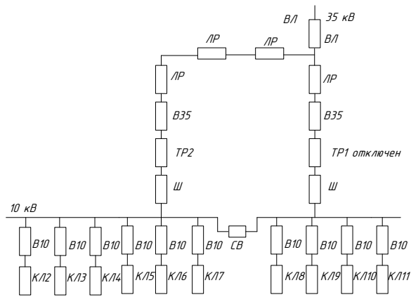
Рисунок 9 - Схема замещения до реконструкции
