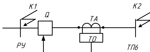
Рисунок 10 - Расчетная схема
