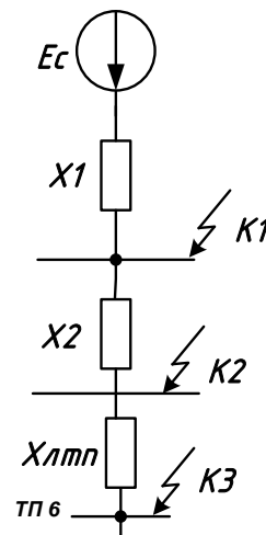
Рисунок 4 - Преобразование схемы замещения на шинах 10 кВ
