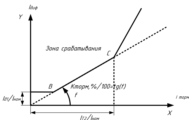
Рисунок 12 - Тормозная характеристика дифференциальной защиты
