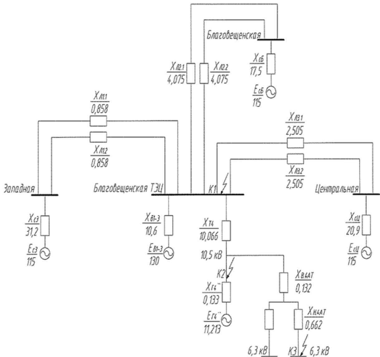
Рисунок 1.2 - Схема замещения прямой последовательности
