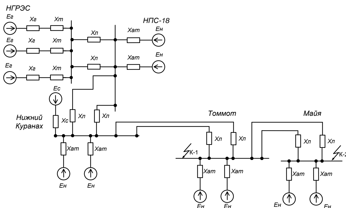
Рисунок 7 – Схема замещения прямой последовательности
