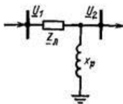
Рисунок 14 - Схема замещения реактора, включенного в линию
