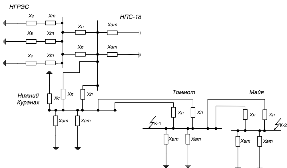
Рисунок 12 – Схема замещения нулевой последовательности
