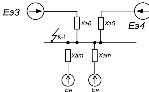
Рисунок 9 – Результирующая схема замещения прямой последовательности
