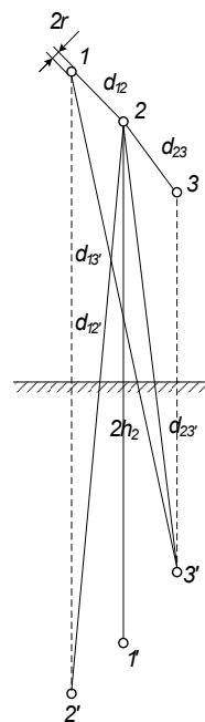
Рисунок 16 – К расчету волновых сопротивлений проводов и тросов
