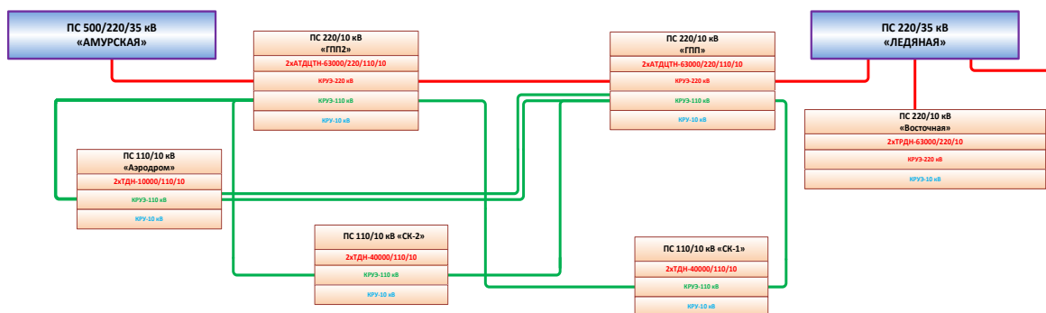
Рис. 2. Блок-схема внешнего электроснабжения космодрома Восточный на 2022 год.
