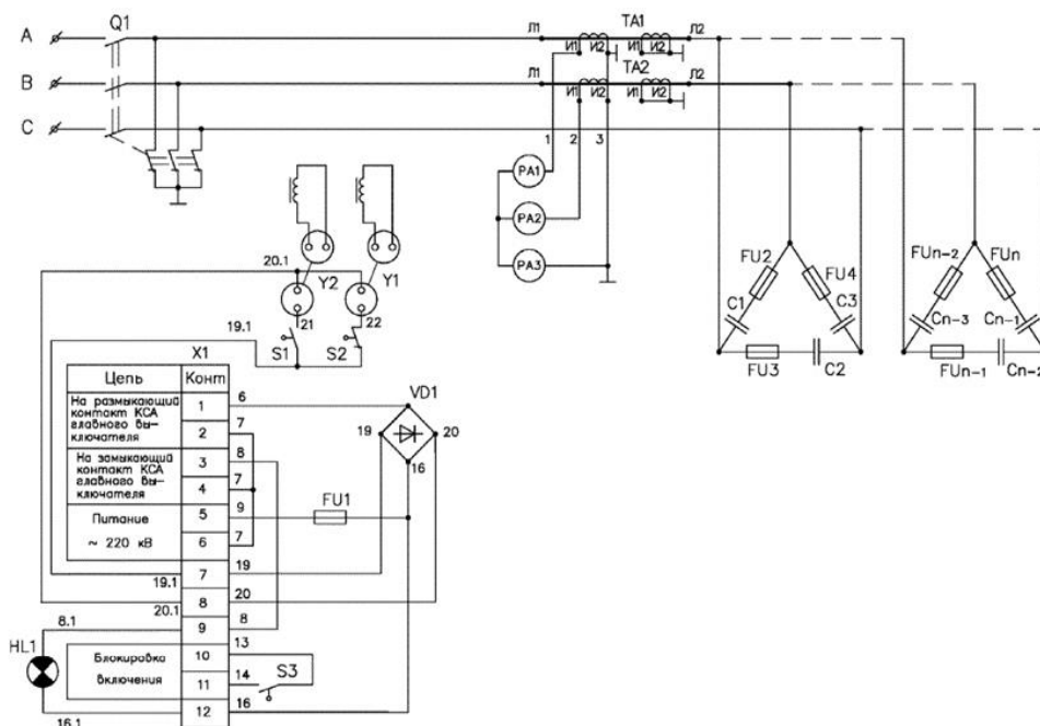
Рис. 3. Однолинейная схема компенсаторной установки
