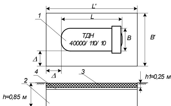
Рис. 12. Схема маслоприёмника
