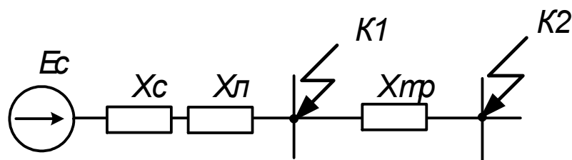
Рис. 4. Схема замещения прямой последовательности
