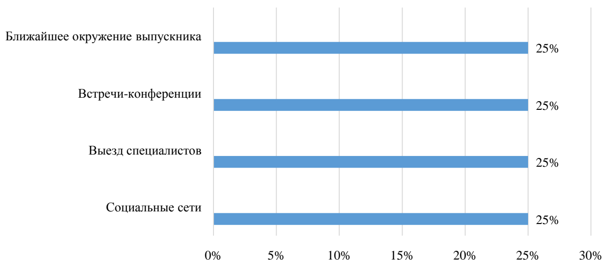
Рисунок 10 – Вида коммуникаций
