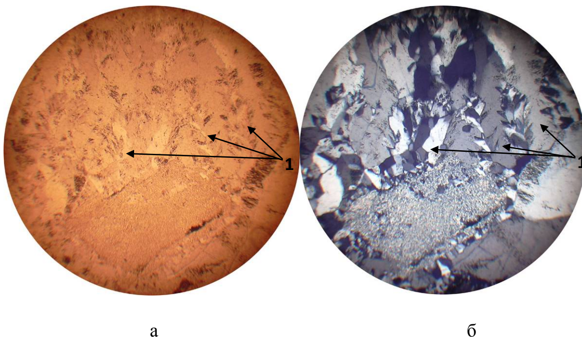
Рисунок 5 – вытянутые листоватые зерна кварца 1 между крупными зернами. Диорит-порфирит. Прозрачный шлиф; а - // николи, б – Х николи. Увеличение 50 x .
