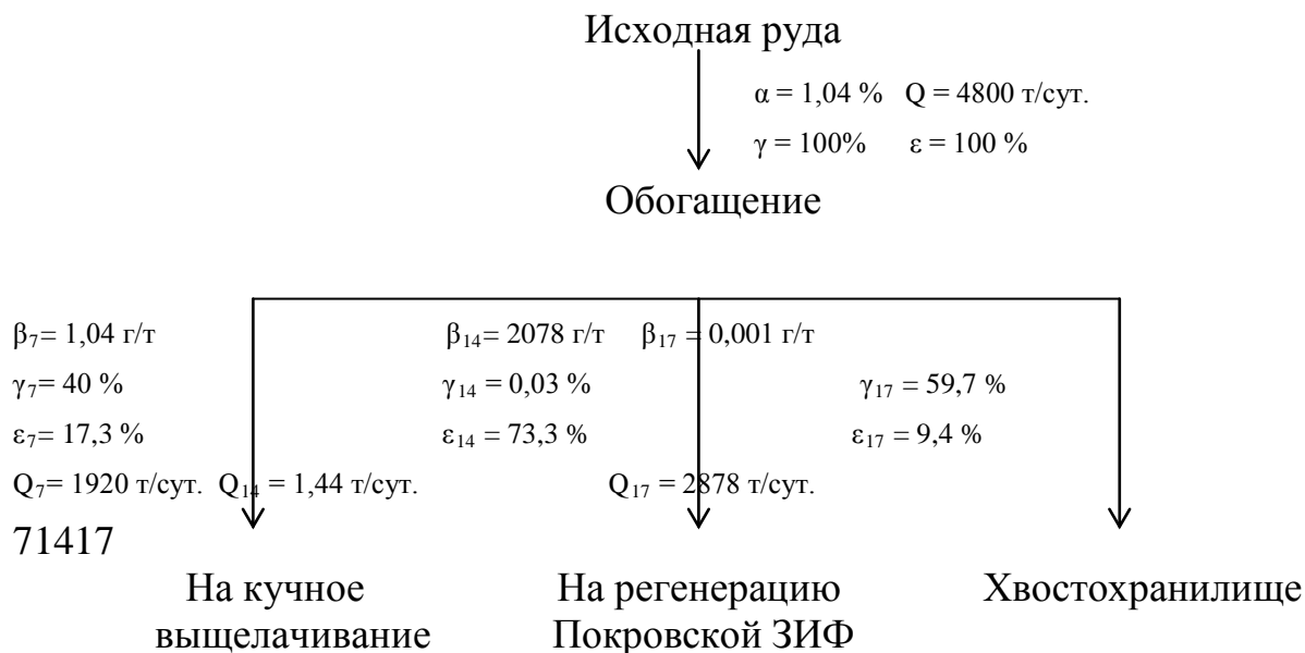
Рисунок 10 – Технологическая схема для расчета основного баланса металлов
