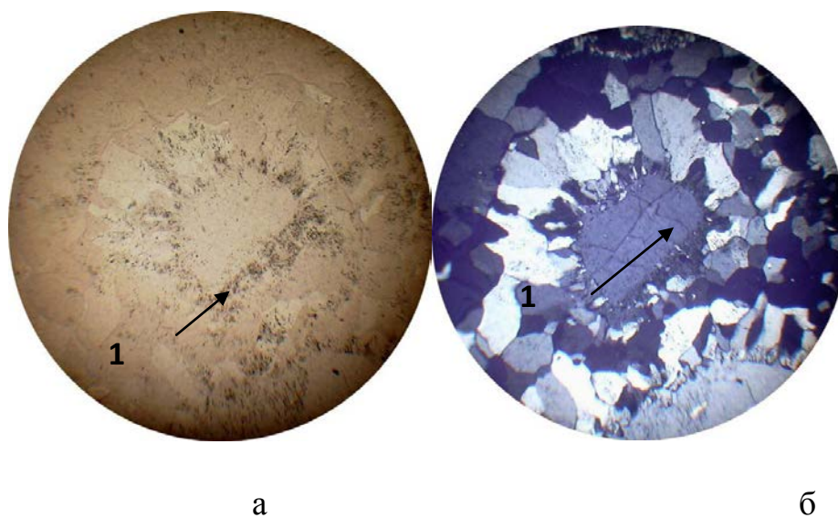
Рисунок 4 – Крупное зерно кварца 1 в ореоле мелких остроконечных зерен. Диорит-порфирит. Прозрачный шлиф; а - // николи, б – Х николи. Увеличение 50 х .
