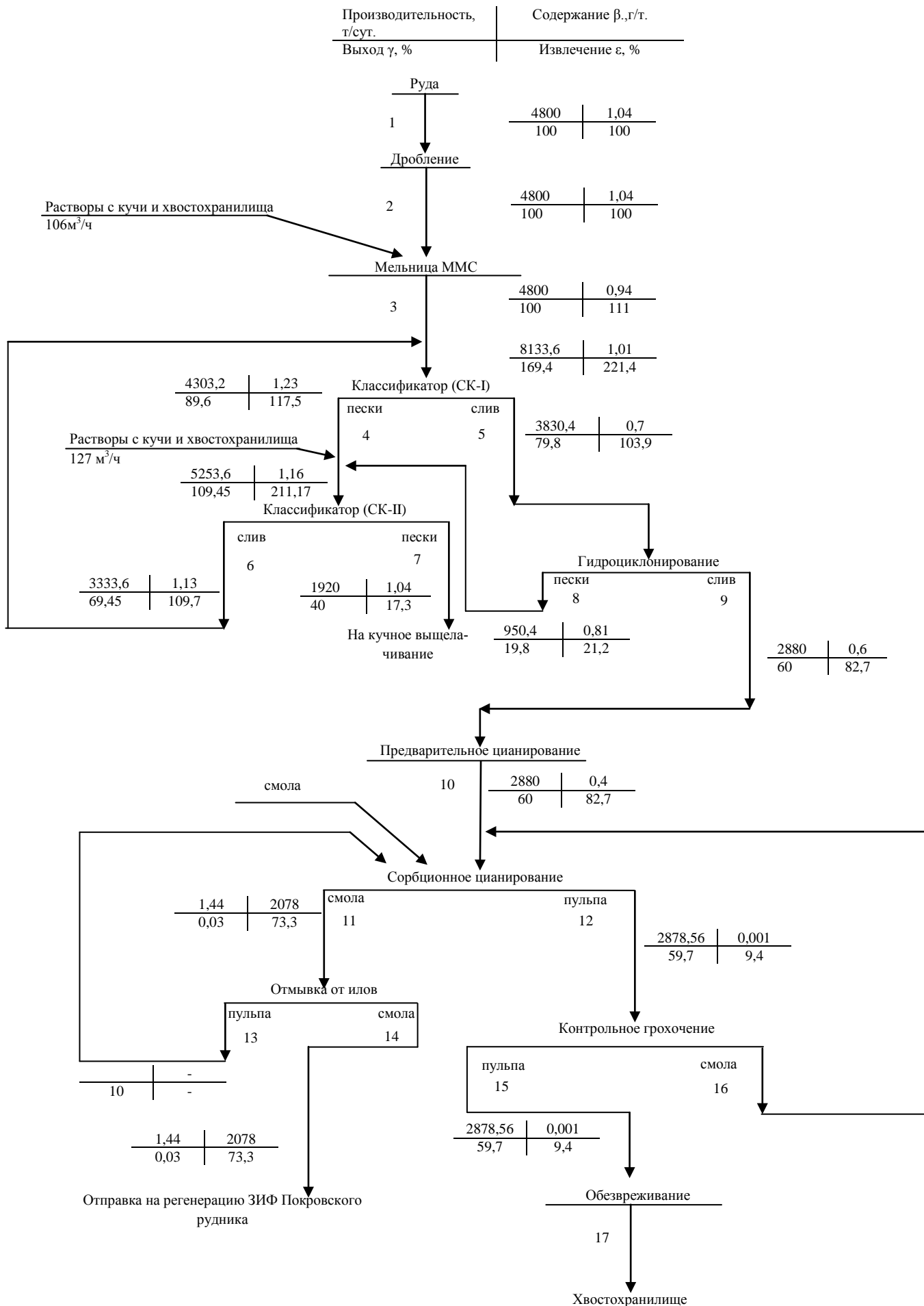
Рисунок 9 – Основная схема обогащения 26
