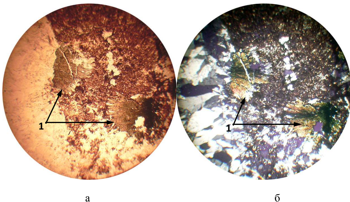
Рисунок 3 – Выделения листочков слюды 1 в основной массе разнозернистого кварца. Диорит порфирит. Прозрачный шлиф; а - // николи, б – Х николи. Увеличение 50 х .
