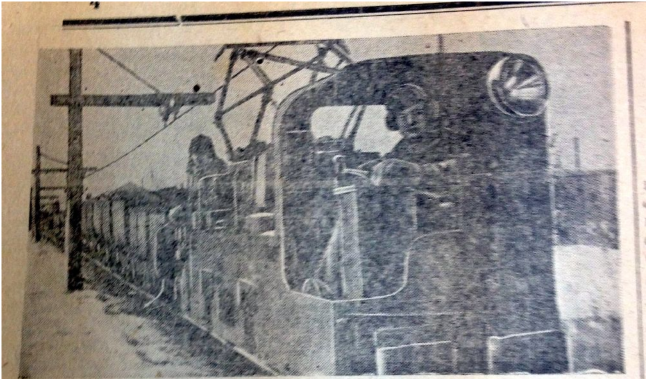
Вывозка угля электровозом по электрифицированной железной дороге со штольни на эстакаду на Кивдинских угольных копях, Бурейнского района, Хабаровского края.
