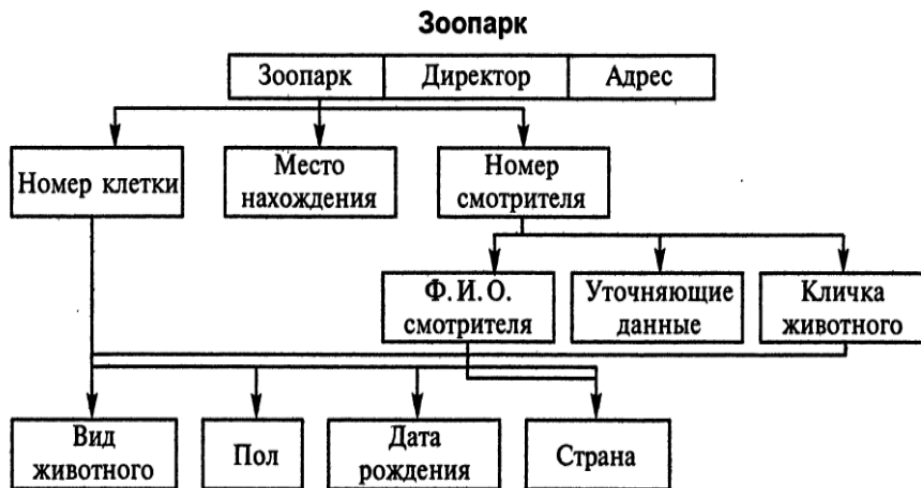
Рисунок 3. Схематическое представление сетевой модели
