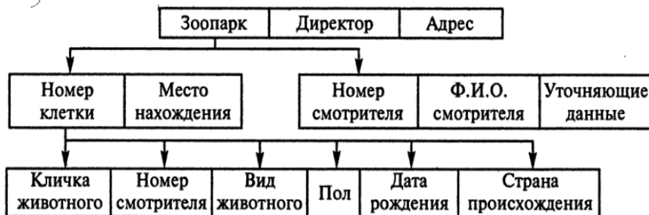
Рисунок 4. Преобразование сетевой модели в иерархическую
