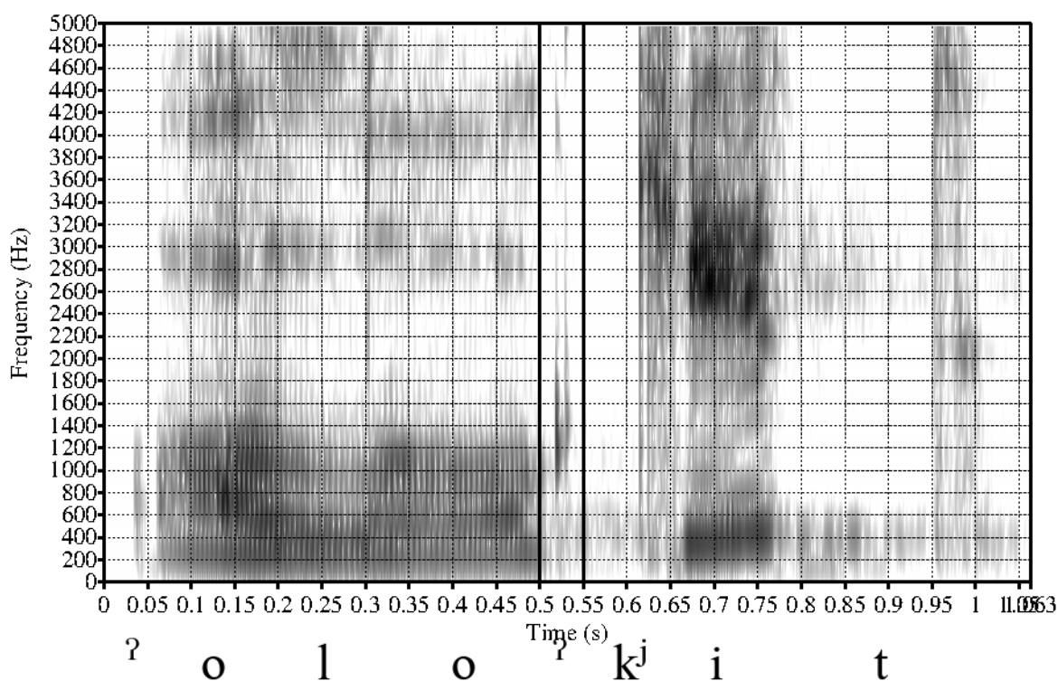
Рис. 10. Поствокальный шум в слове олокит (= брод)
