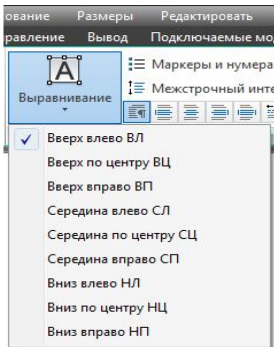
Рис. 6.11. Подменю Выравнивание .
