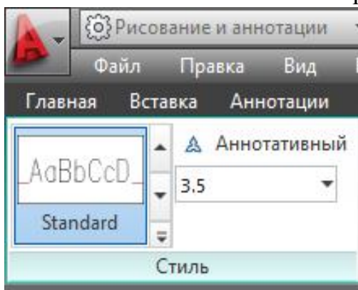
Рис. 6.10. Панель Стиль .
