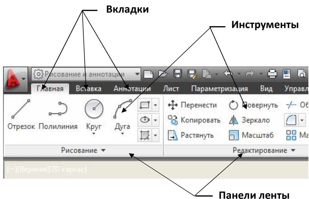
Рис.1.4. Элементы ленты.
