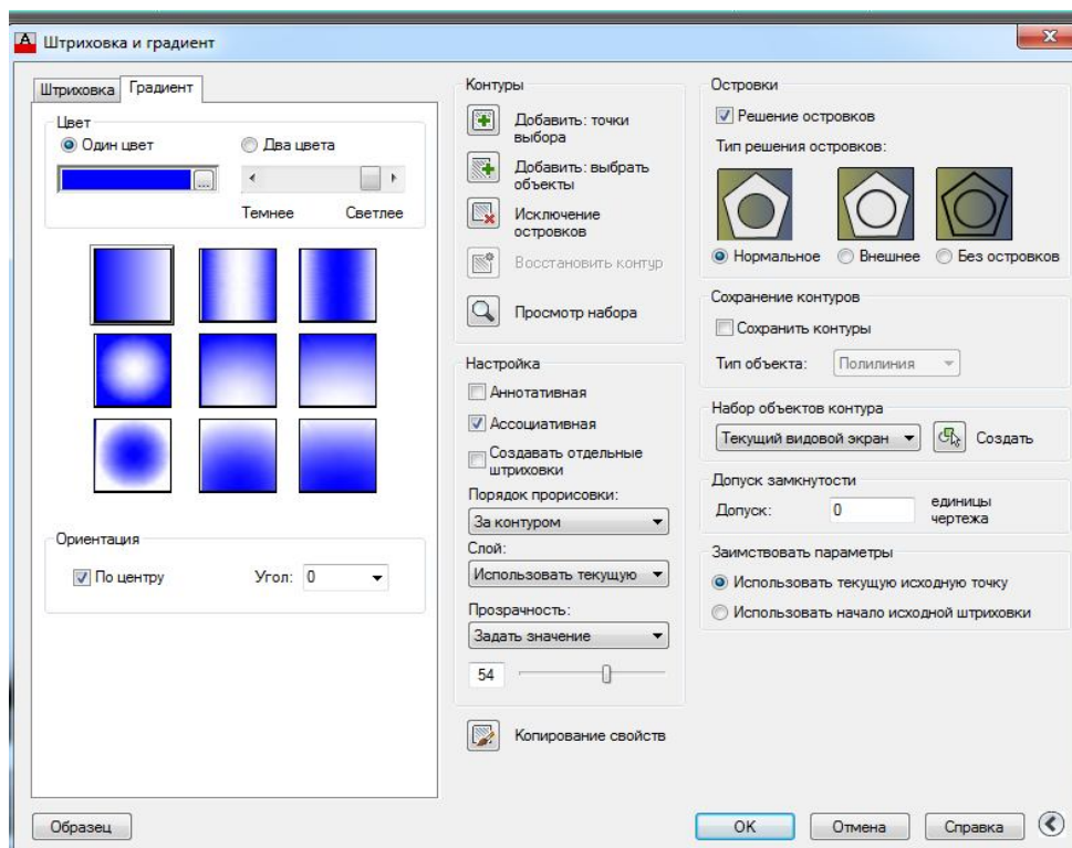
Рис. 3.17. Вкладка Градиент .
