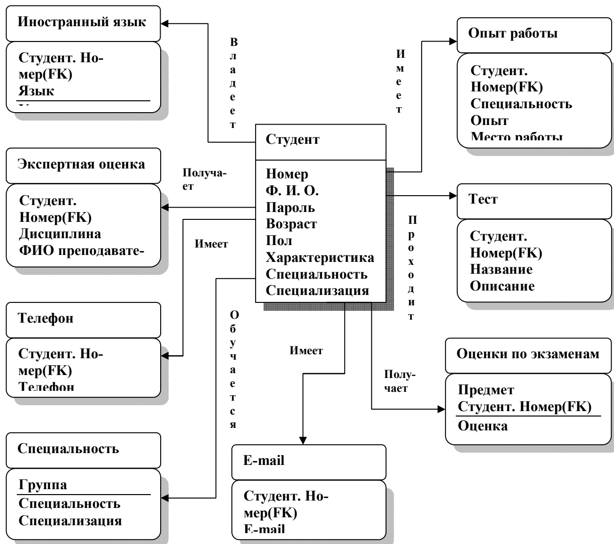
ERD-диаграмма БД студентов в третьей нормальной форме
