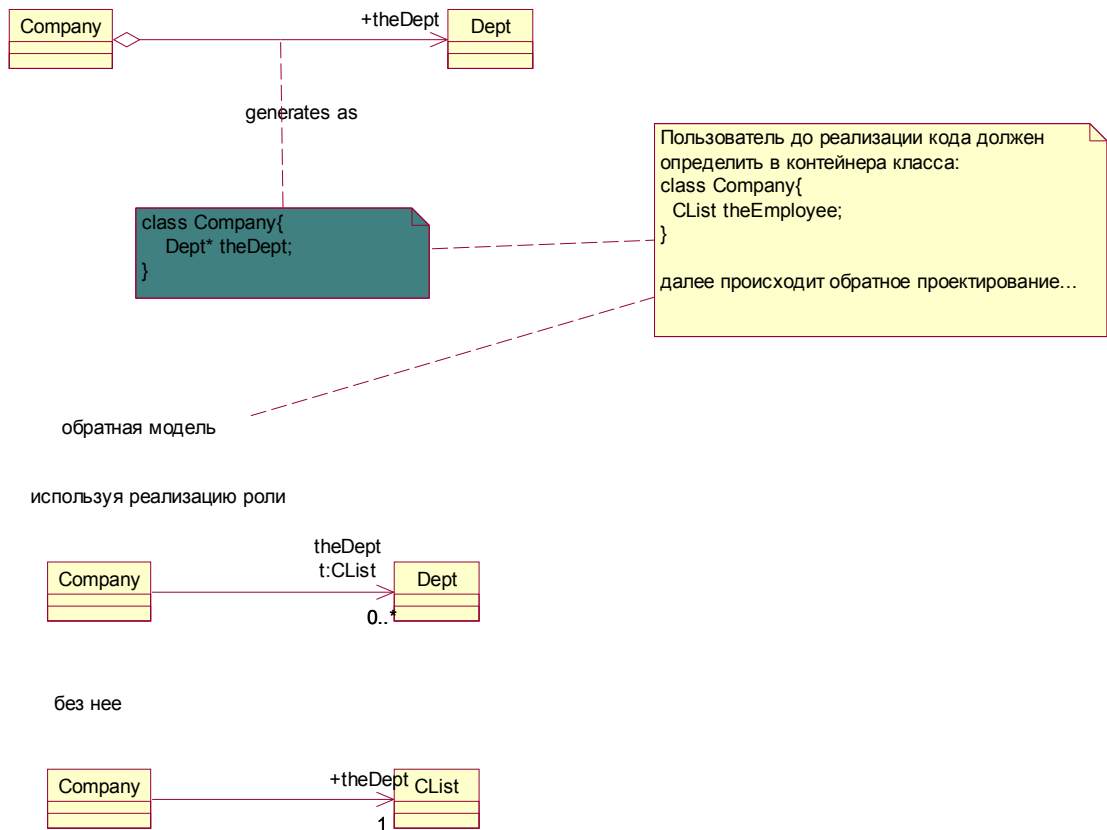
Рис.24. Сохранение первоначальной семантики проекта.
