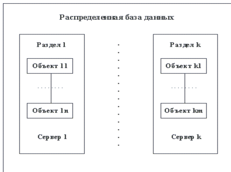
Рис. 1.3. Распределенная база данных с логически автономными разделами
