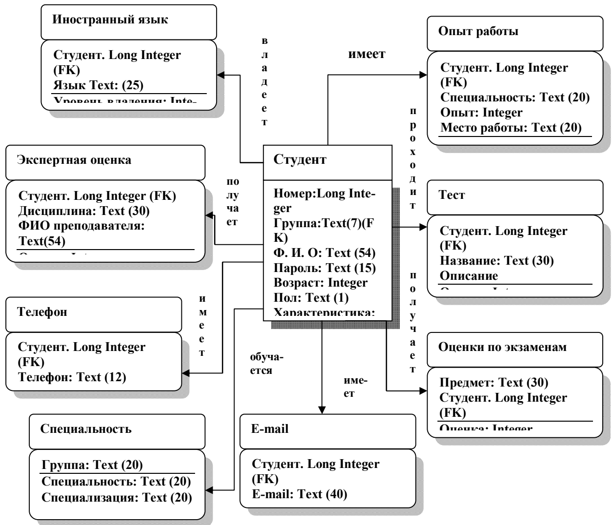
Скорректированная физическая модель БД студентов
