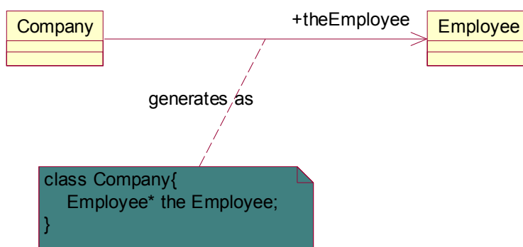
Рис.21. Простая ассоциация.
