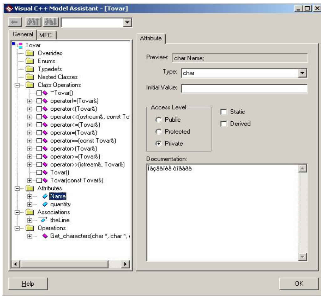
Рис.16. Редактирование атрибутов класса при помощи Model Assistant.
