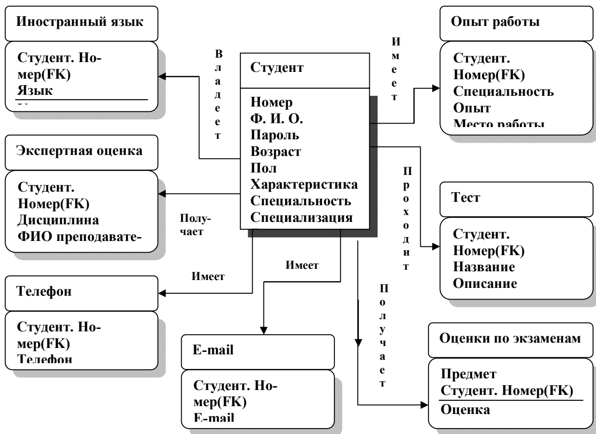
ERD-диаграмма БД студентов в первой нормальной форме
