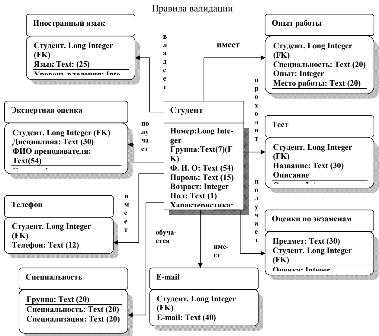
Физическая модель БД студентов
