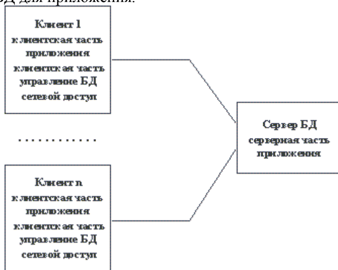
Общее представление информационной системы
