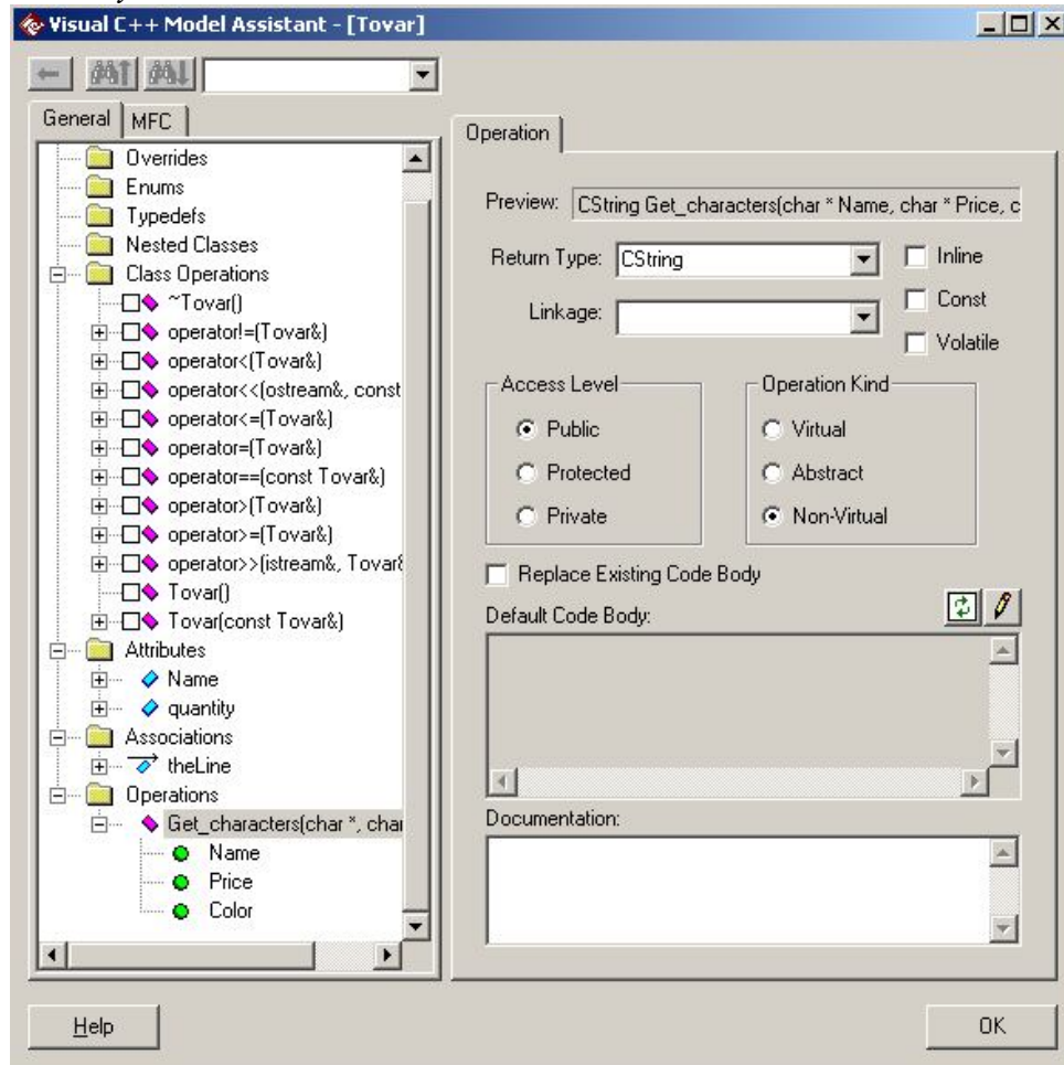
Рис.15. Свойства операции Get_characters .
