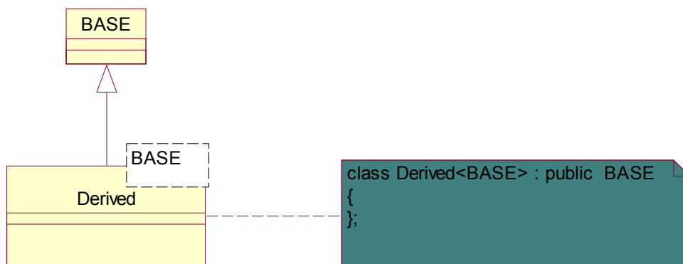
Рис.19. Определение класса Шаблона.
