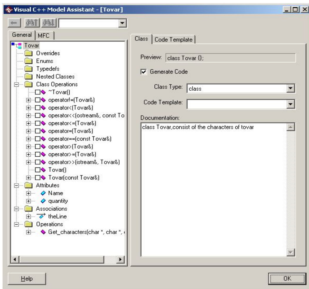
Рис.14. Model Assistant для класса Tovar.
