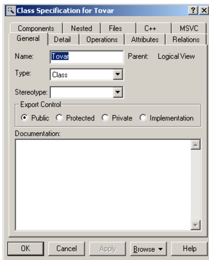
Рис.4. Окно свойств класса Товар.
