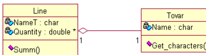
Рис. 7. Связь между двумя классами.
