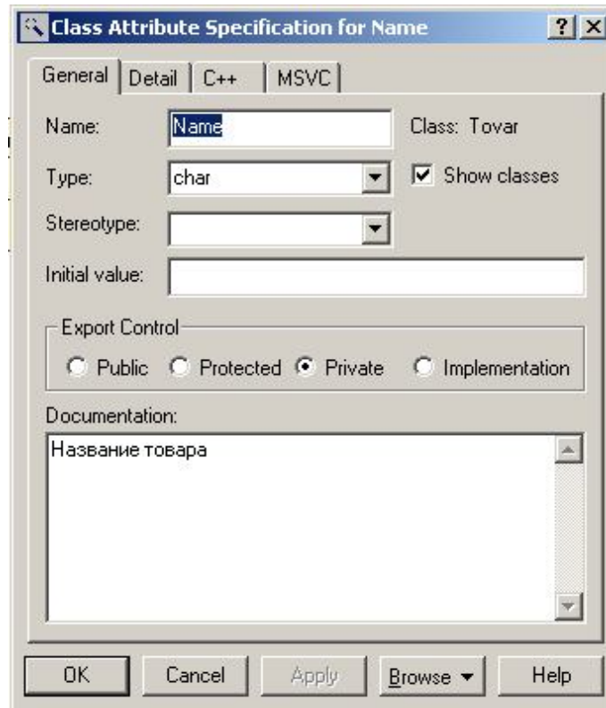
Рис.5. Окно свойств атрибута класса.
