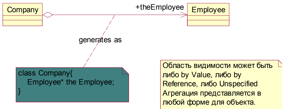
Рис.22. Простая агрегация.
