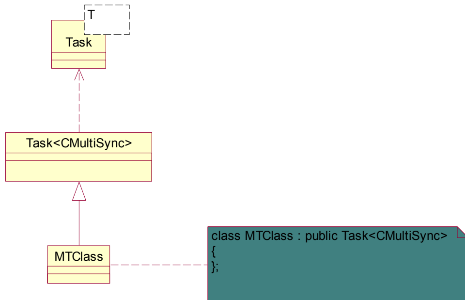
Рис.20. Иллюстрация Шаблона.
