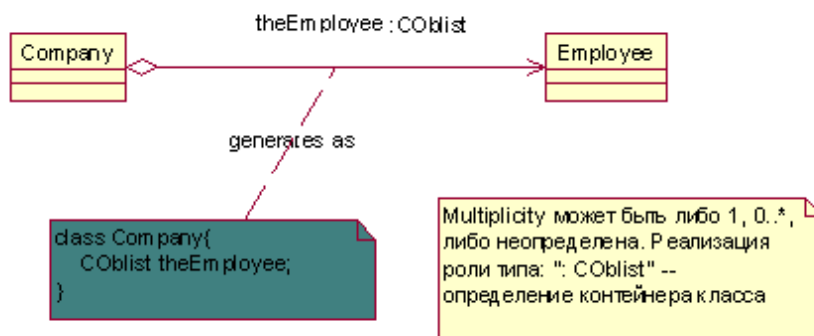
Рис.23. Контейнер класса.
