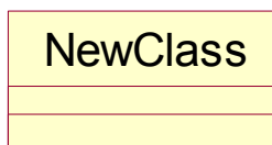
Рис.3. Изображение класса.
