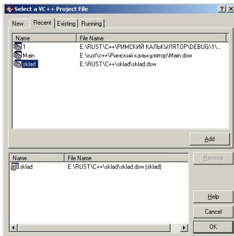
Рис.12. Выбор проекта.
