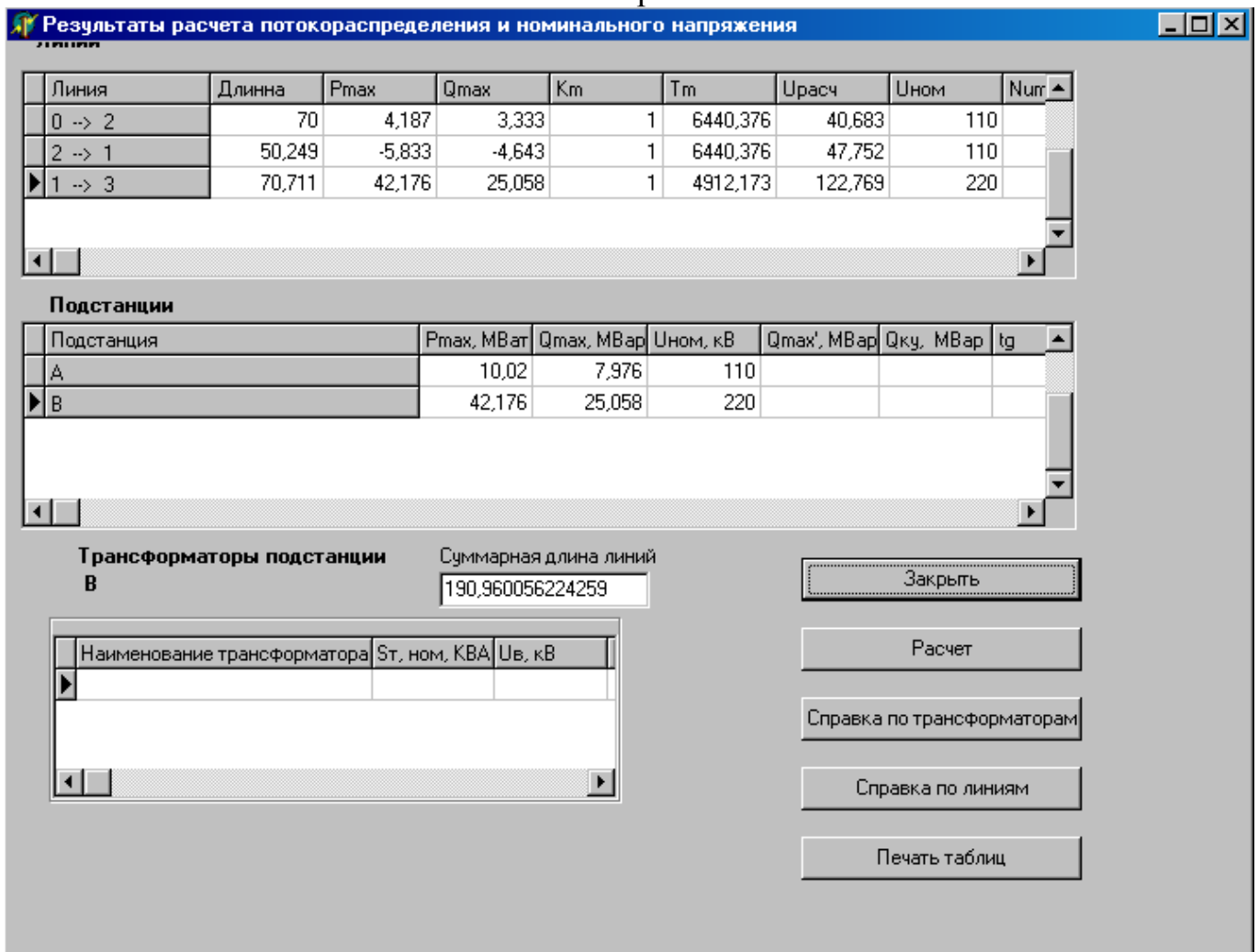
Рис. 28. Результаты расчетов потокораспределения и выбора номинального напряжения
