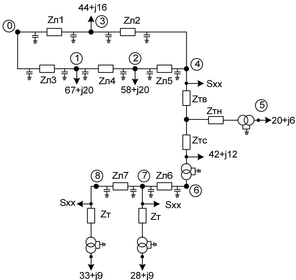
Рис. 2. Схема замещения электрической сети.
