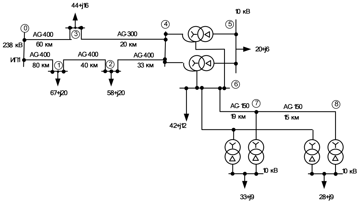
Рис. 1. Электрическая схема сети.
