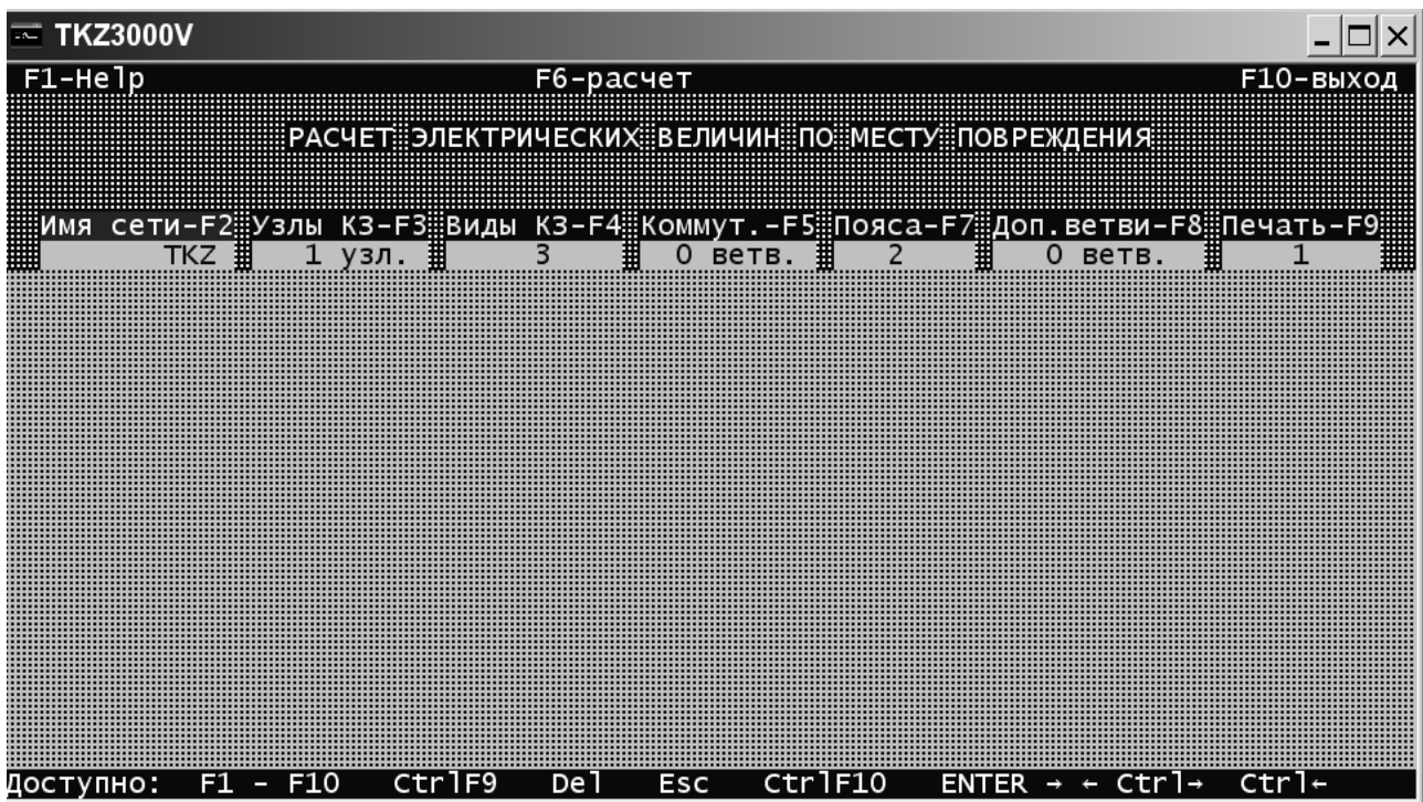
Рис. 21. Окно расчета переходных электромагнитных процессов в программе TKZ.
