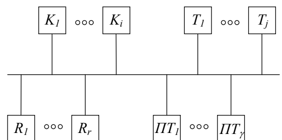
Рис. 3. Схема энергосистемы:
