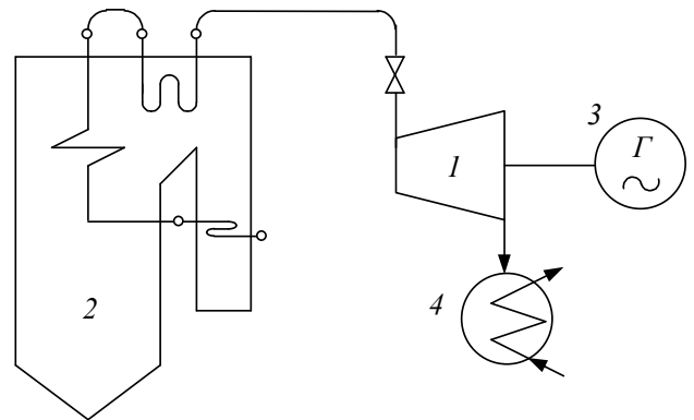
Рис. 4. Схема энергоблока:
