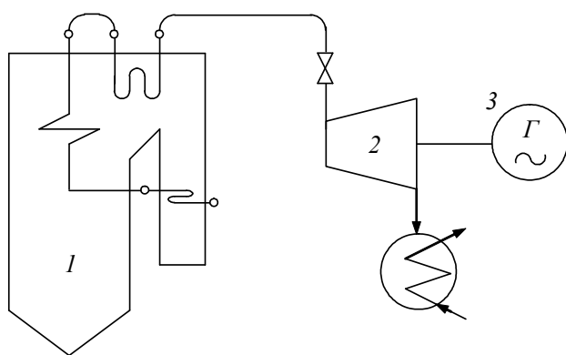
Рис. 5. Схема последовательных соединений элементов: 1 – котел, 2 – турбина, 3 – электрогенератор
