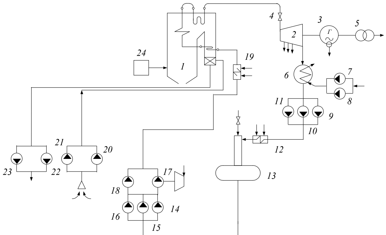
Рис. 5. Расчетная тепловая схема энергоблока Исходные данные и расчетные показатели надежности
