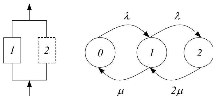
Рис. 1. Схема и граф состояний с ненагруженным резервом:
