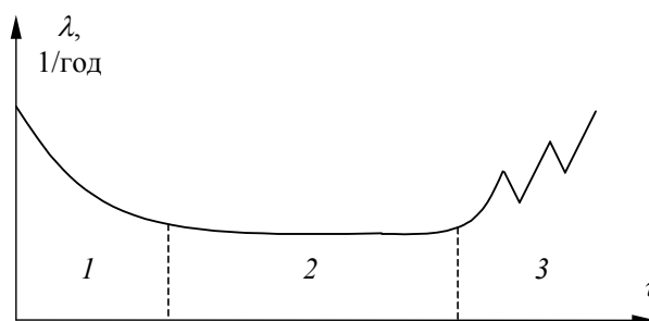
Рис. 3. Интенсивность отказов за период жизни элемента
