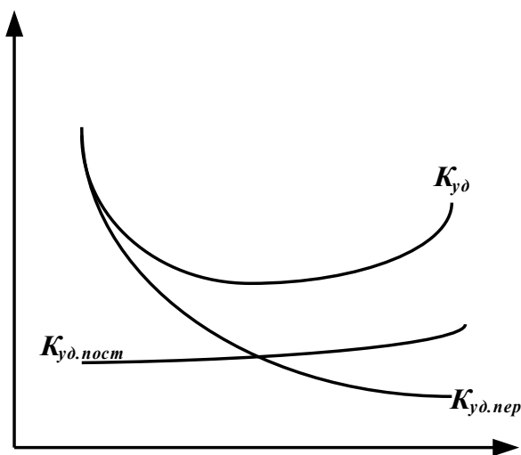
Рис. 15. Зависимость удельных капиталовложений от мощности оборудования электростанции
